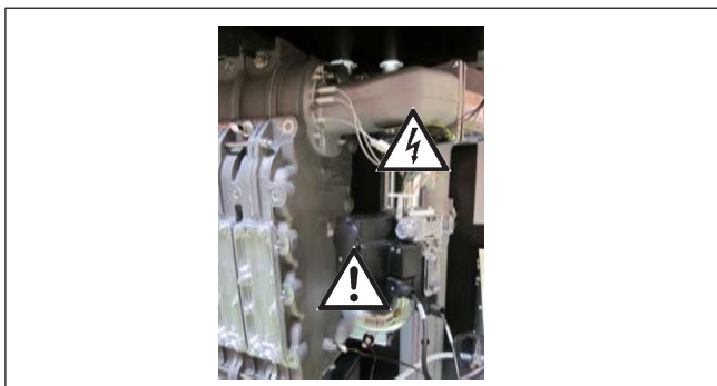
Bild: Zündtrafo, Hochspannungs-Zündeletrode, Gaskombiventil, Gasdruckwächter, Ventilator, Brennkammer Gefahr durch elektrische Spannung, Gefahr von Vergiftung und Explosion durch ausströmendes Gas, Gefahr von Verbrennung durch heiße Bauteile.
