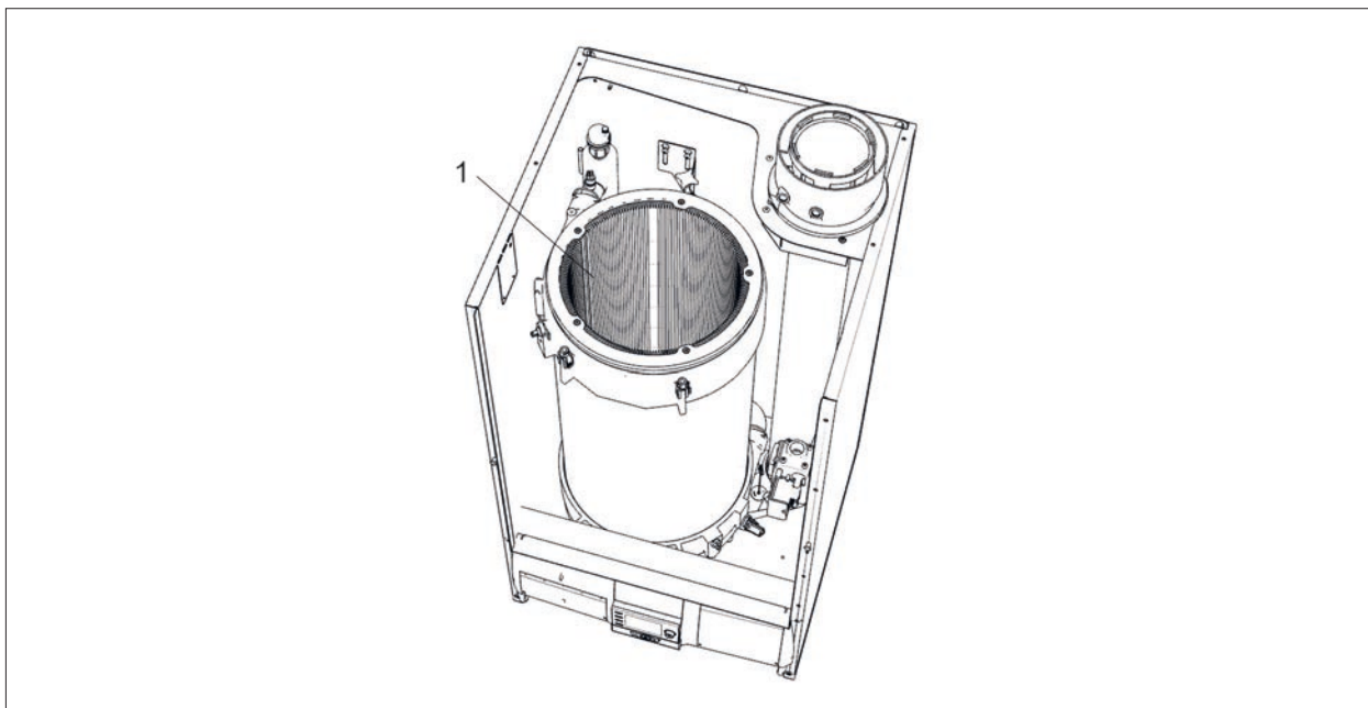
Abb. 6.8 Wärmetauscher reinigen
