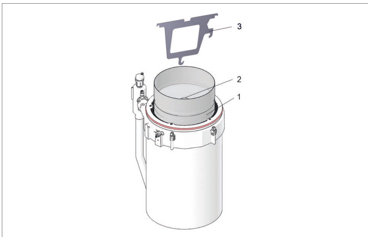
Abb. 6.6 Brennkammertopf ausbauen
