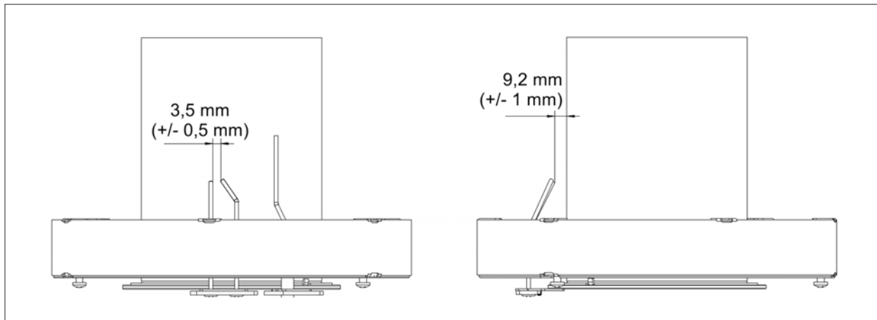
Abb. 6.5 Abstände Zündelektrode
