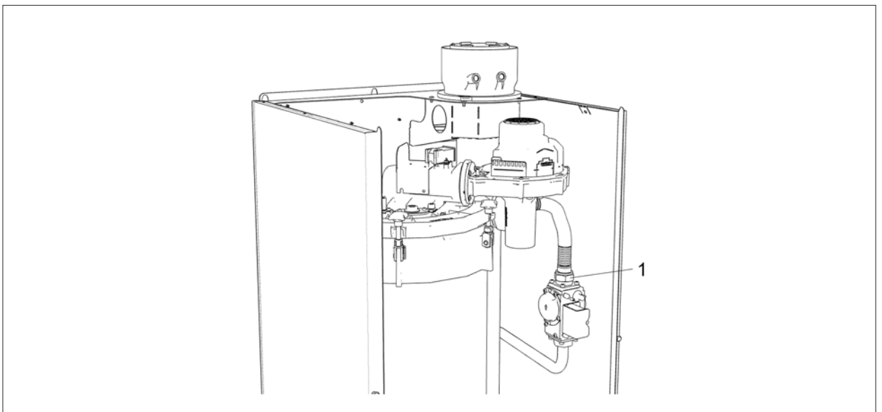
Abb. 5.4 Gasleitung öffnen
