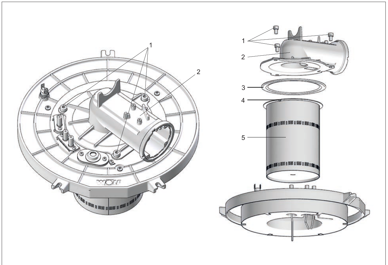
Abb. 6.2 Brenner zerlegen
