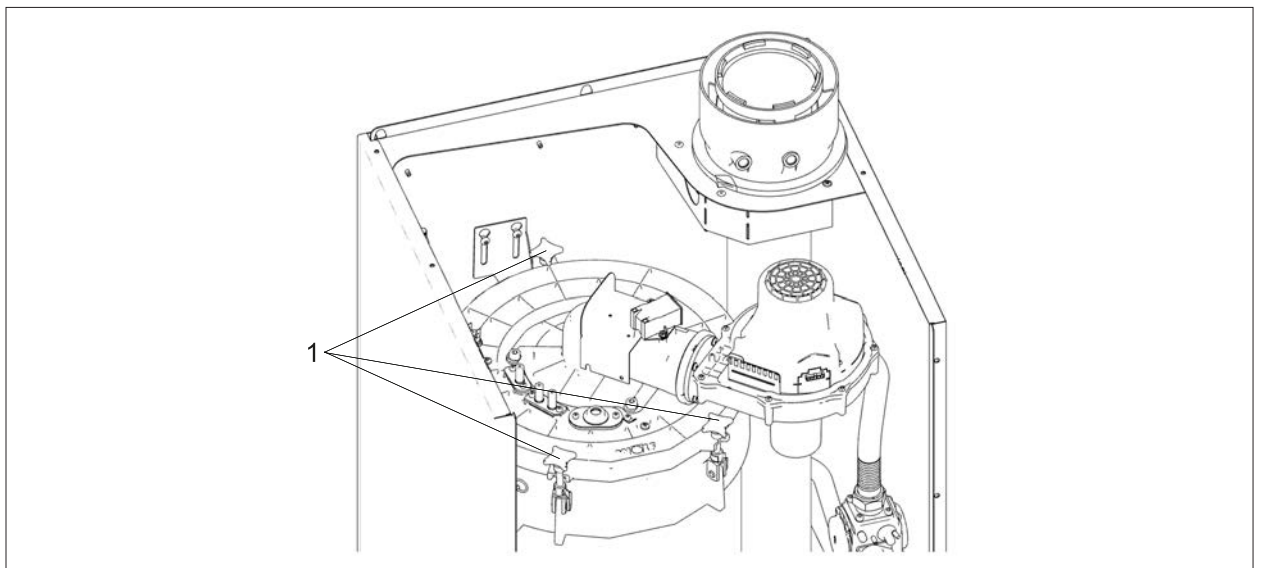
Abb. 6.10 Brennkammerdeckel montieren
