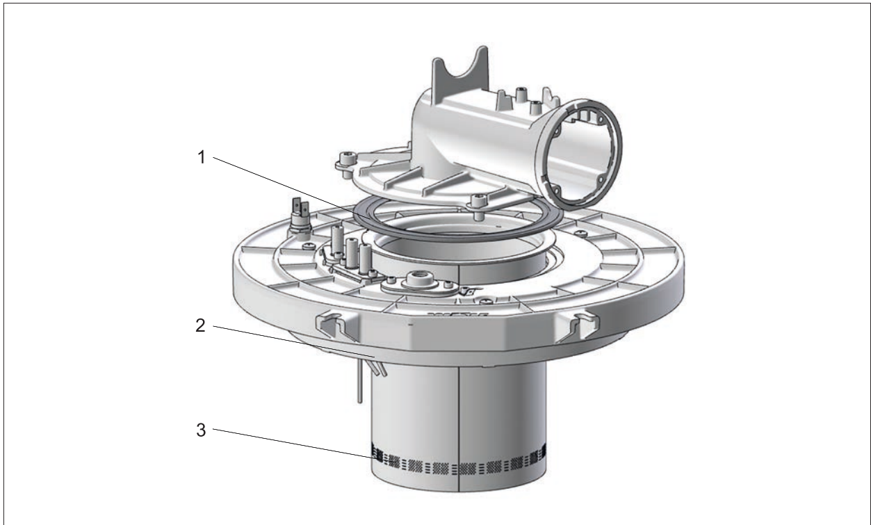
Abb. 6.1 Sichtkontrolle Brenner
