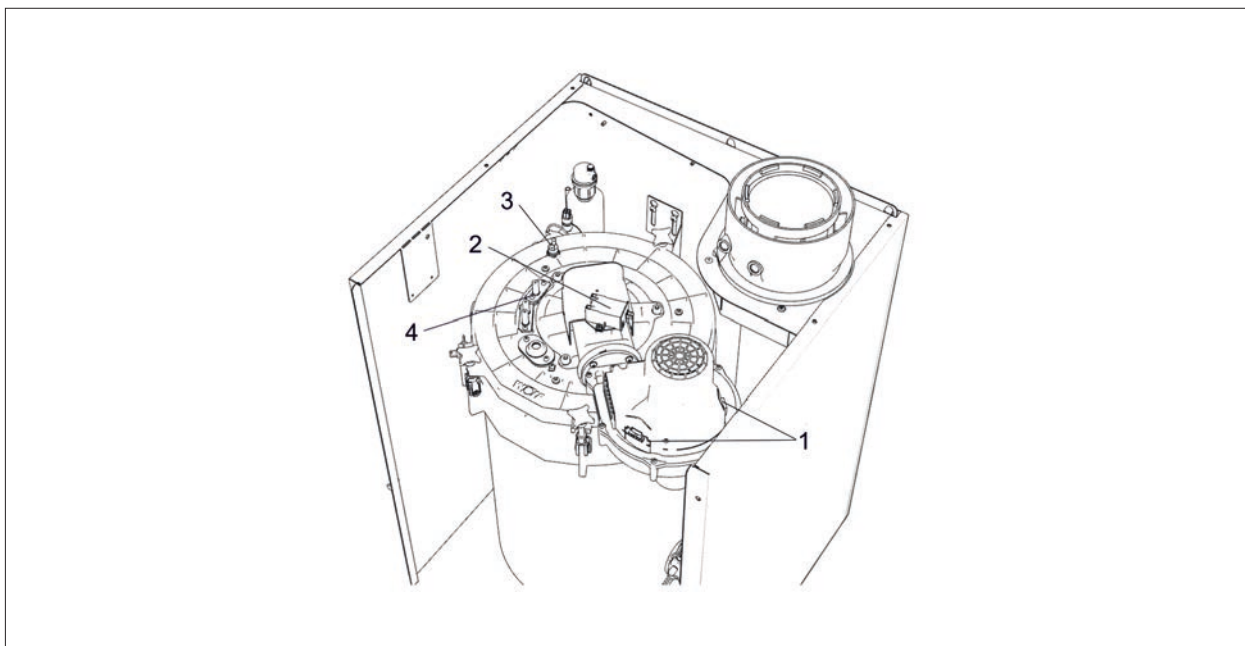
Abb. 5.5 Anschlusskabel Brenner lösen
