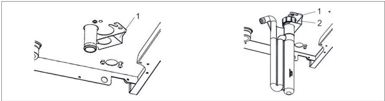
Abb. 6.11 Siphon reinigen
