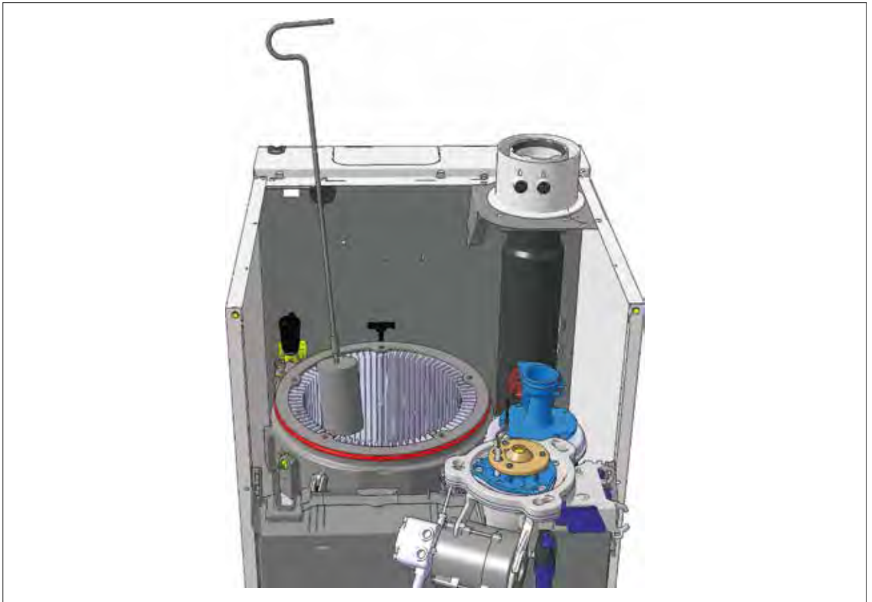
Abb. 4.16 Heizwasserwärmetauscher bürsten
