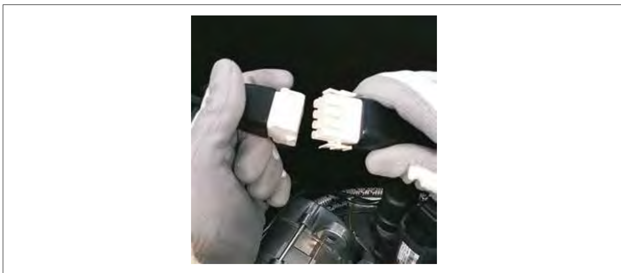
Abb. 4.3 Brennerstecker abziehen
