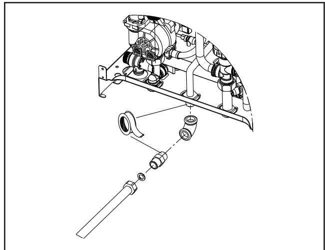
Bild: Montage Gasanschluss
