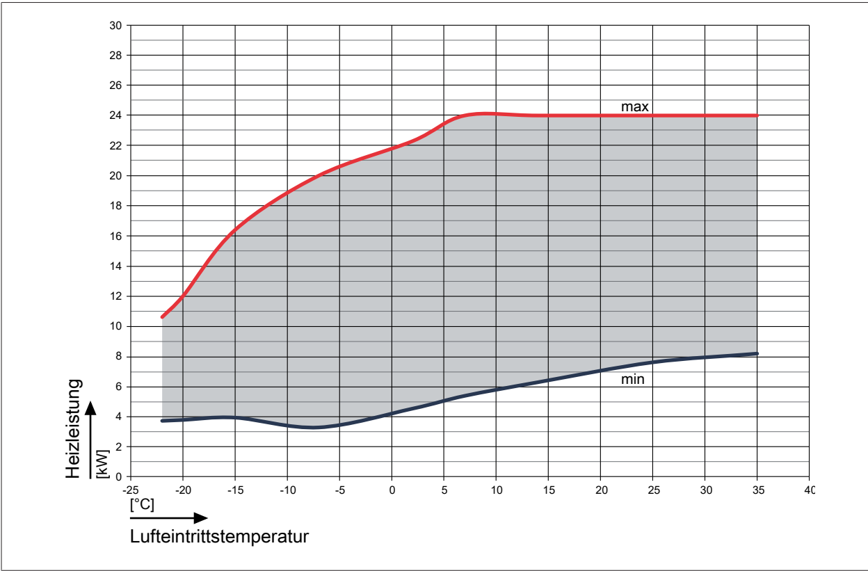
Abb. 5: Heizleistung bei einem Vorlauf von 45 °C
