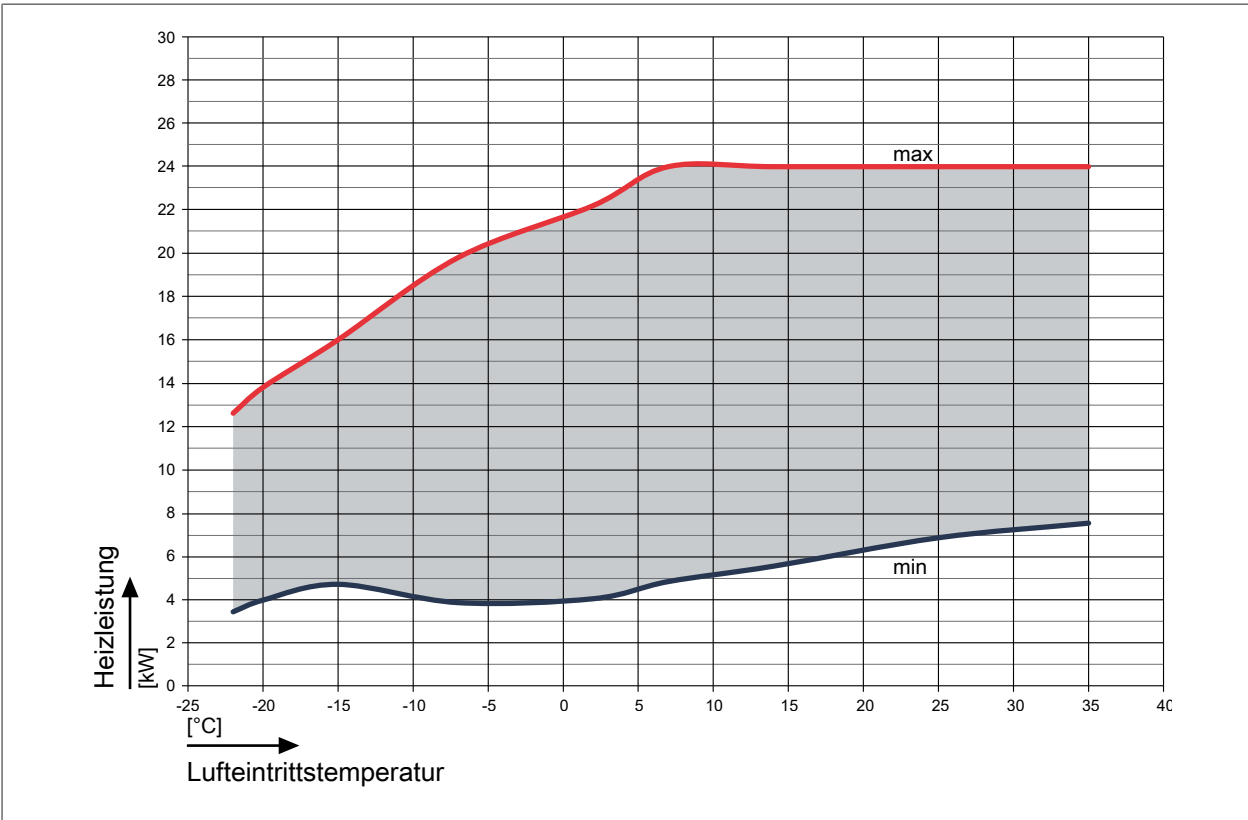
Abb. 6: Heizleistung bei einem Vorlauf von 55 °C
