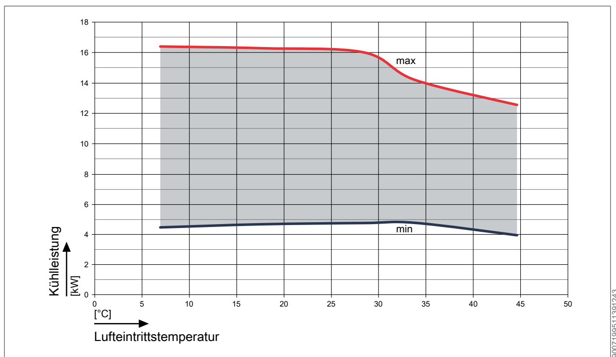
Abb. 9: K hlleistung bei einem Vorlauf von 7  C
