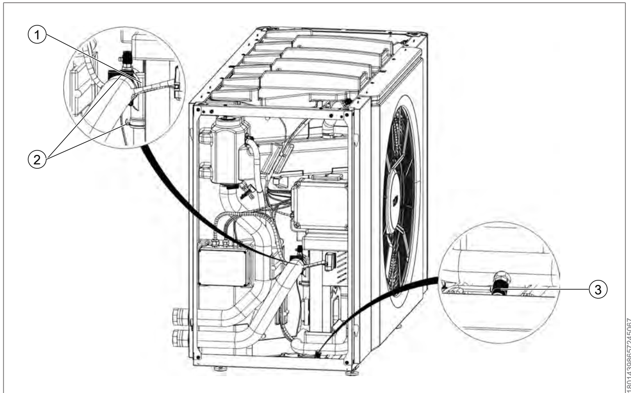
1 Messinggehäuse 3 Entleerungshahn
