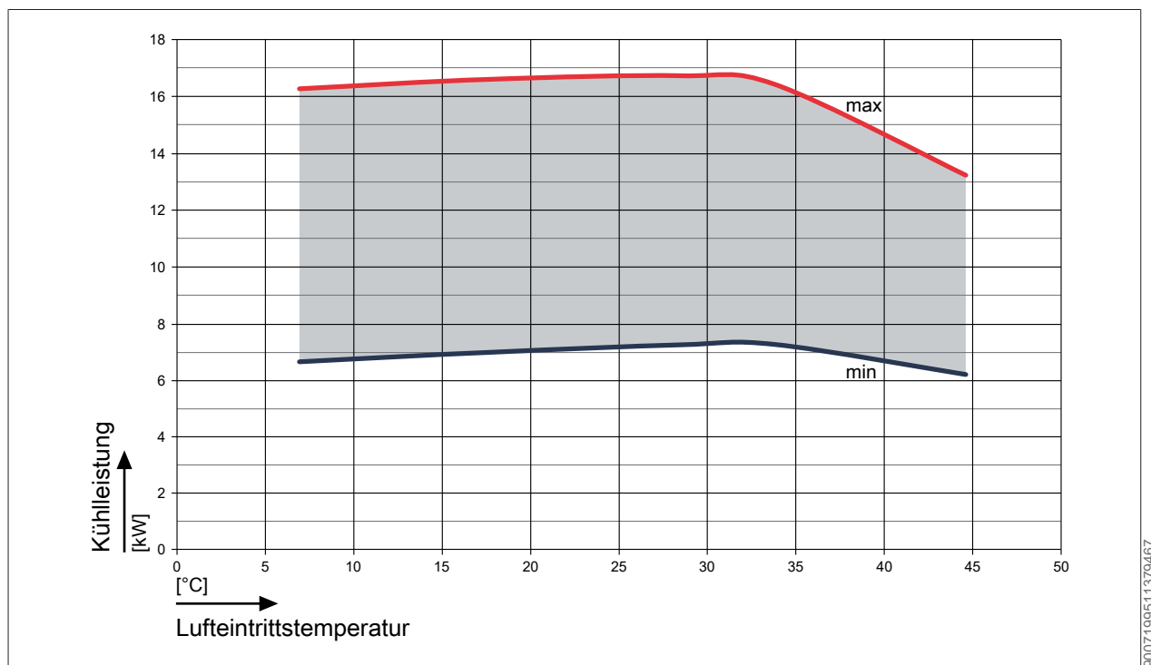
Abb. 8: K hlleistung bei einem Vorlauf von 18  C
