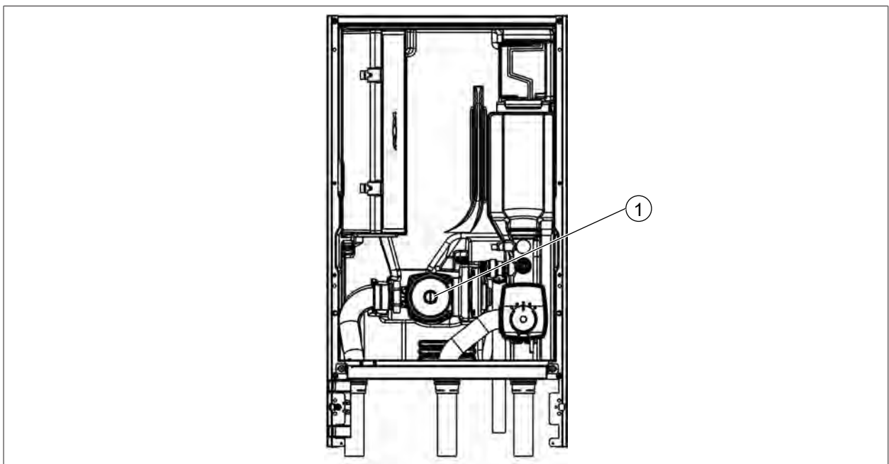
1 Entlüftungsschraube
