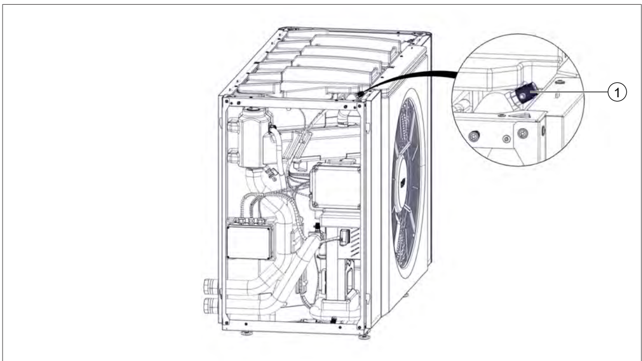
1 Handentlüfter (Luft-/Klätemittelabscheider)
