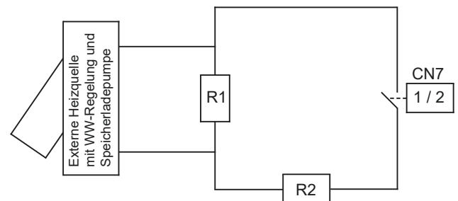
Verdrahtungsplan
