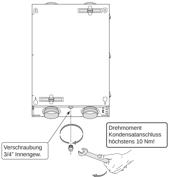
Montage Kondensatablaufstutzen im CWL - F - 150 Excellent (VHZ)
