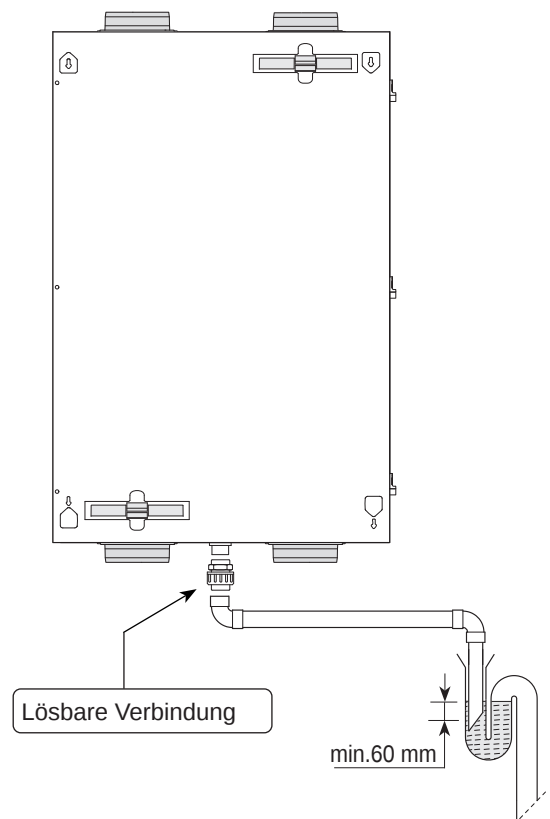
Kondensatablauf bei Wandmontage CWL - F - 150 Excellent (VHZ)
