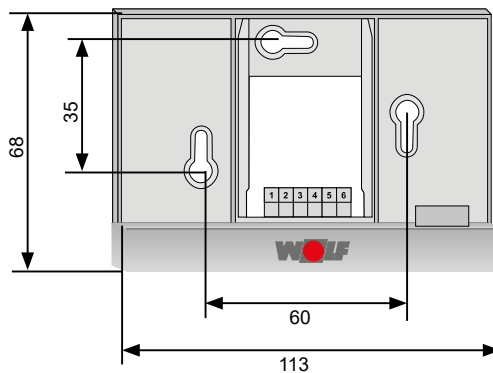
Abb. 4.3 Wandsockel BM-2 Solar mit Schrauben und Dübeln an Wand montieren
