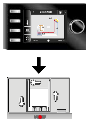
Abb. 4.4 Bedienmodul BM-2 Solar von oben in die Führung am Wandsockel einsetzen
