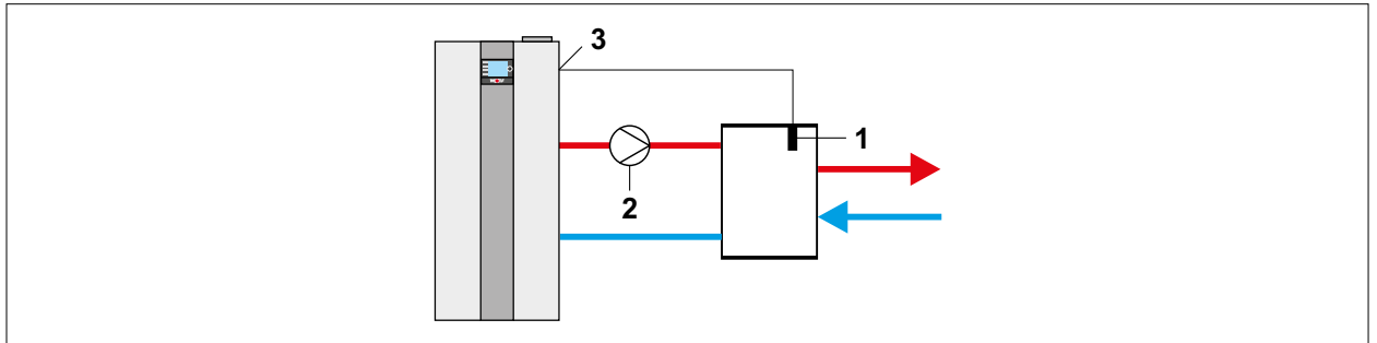
Abb. 13.6 Anlagenkonfiguration 11 - Hydraulische Weiche / Plattenwärmetauscher als Systemtrennung
