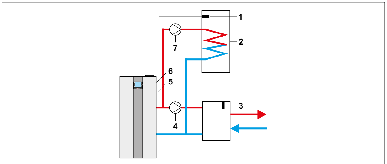
Abb. 13.7 Anlagenkonfiguration 11 - Speicher vor der Hydraulische Weiche / Plattenwärmetauscher als Systemtrennung
