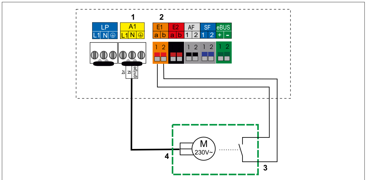
Abb. 13.3 Elektroanschluss Abgasklappe
