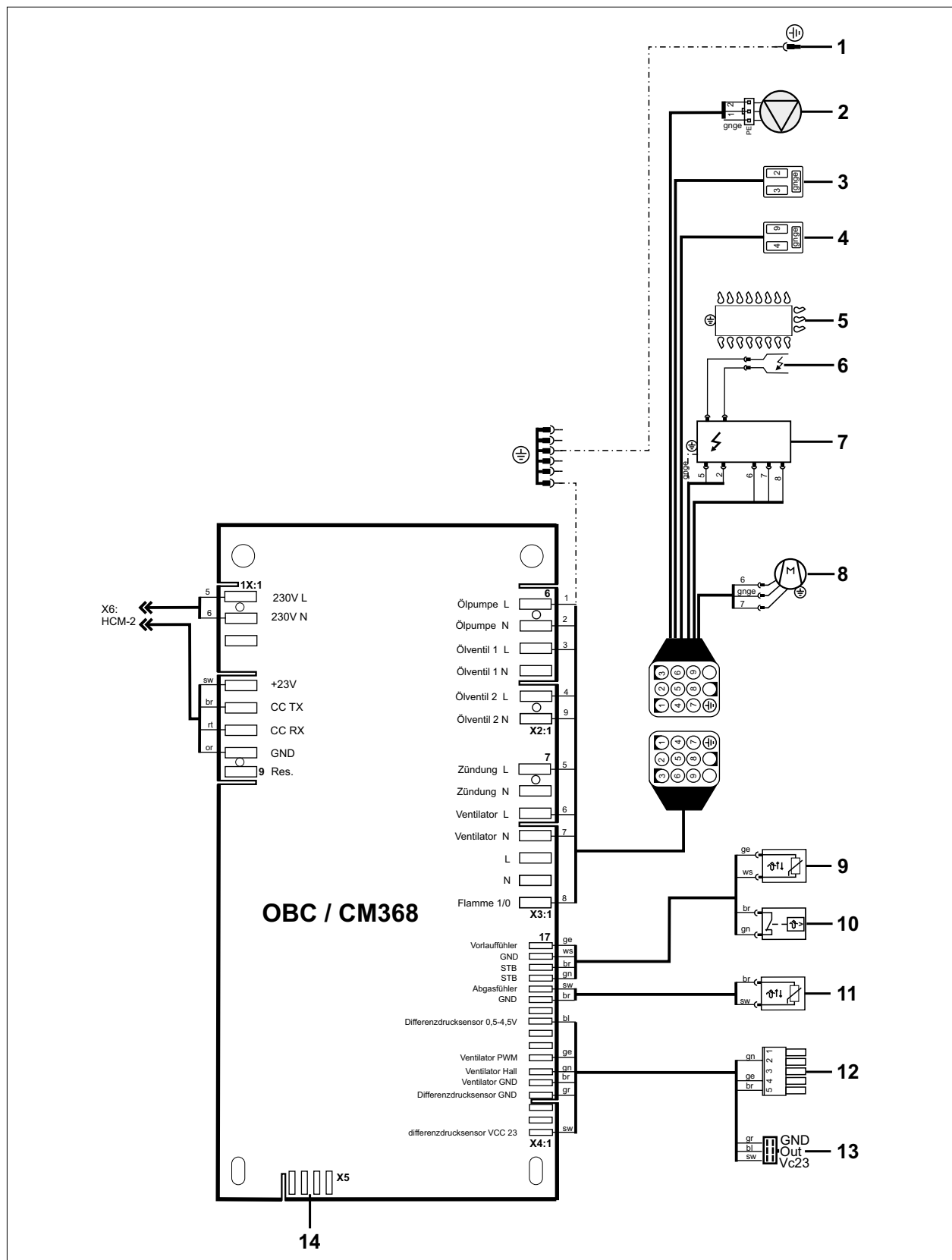
Abb. 13.2 Schaltplan Ölfeuerungsautomat OBC / CM368
