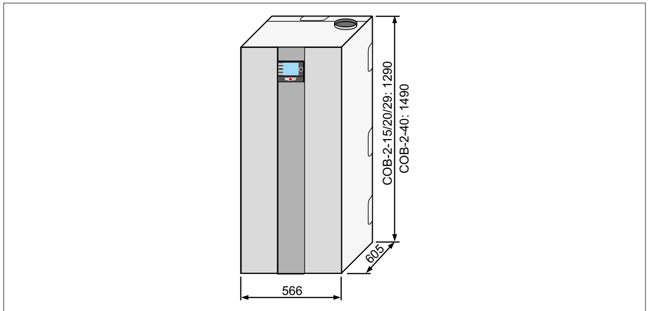
Abb. 12.1 Ölbrennwertkessel COB-2-15/20/29/40 für Heizen mit Anschlussmöglichkeit für Speicherwassererwärmer z. B. SE-2, SEM-..., BSP [mm]
