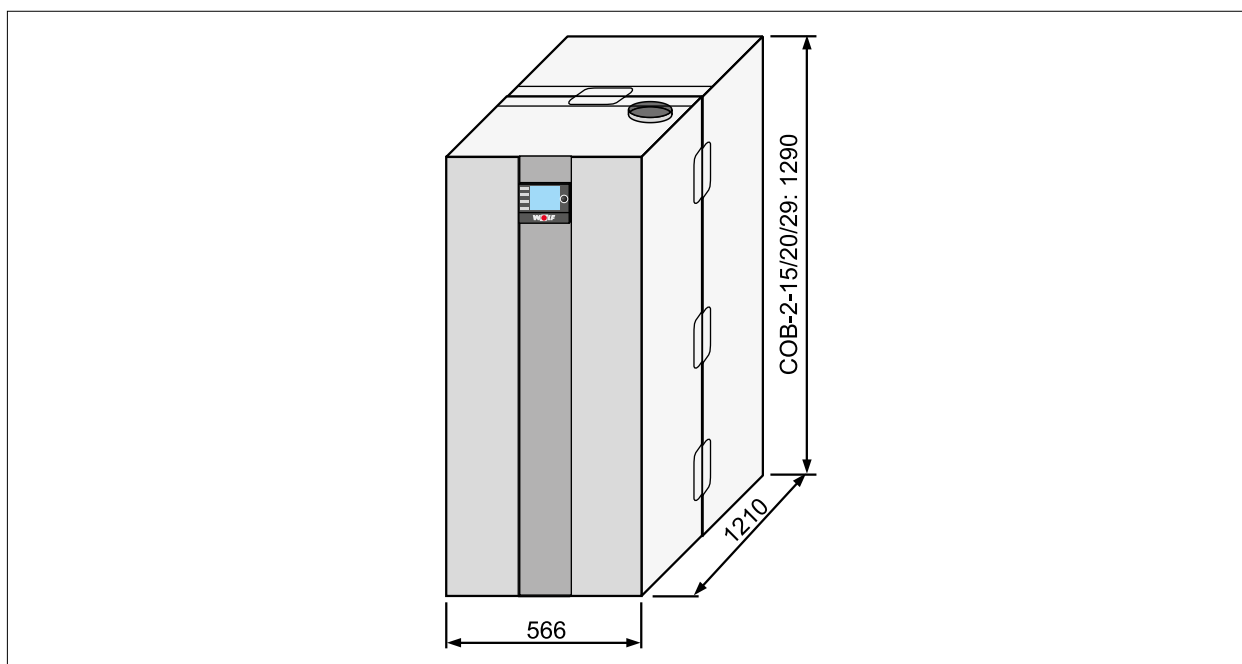
Abb. 12.3 Ölbrennwertkessel COB-2-15/20/29 mit Speicher TS/TR, hinten stehend [mm]
