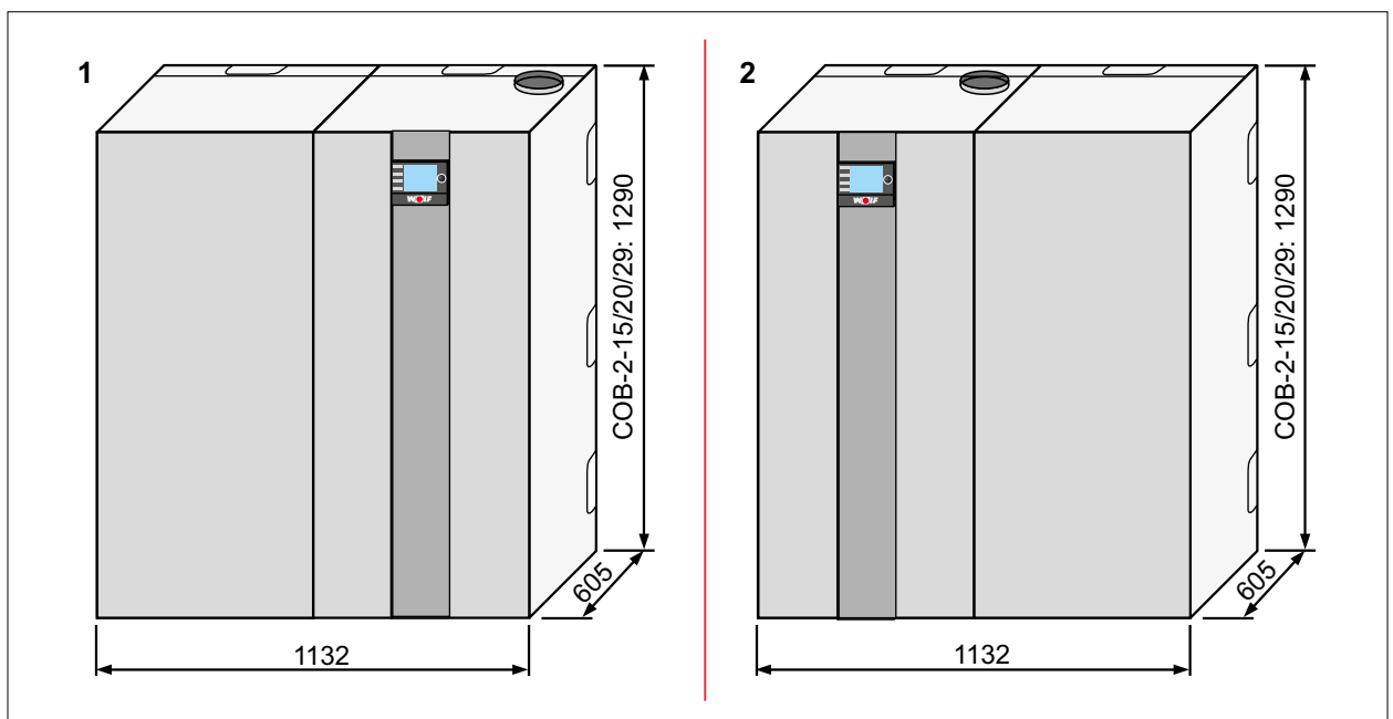
Abb. 12.2 Ölbrennwertkessel COB-2-15/20/29 mit Speicher TS/TR
