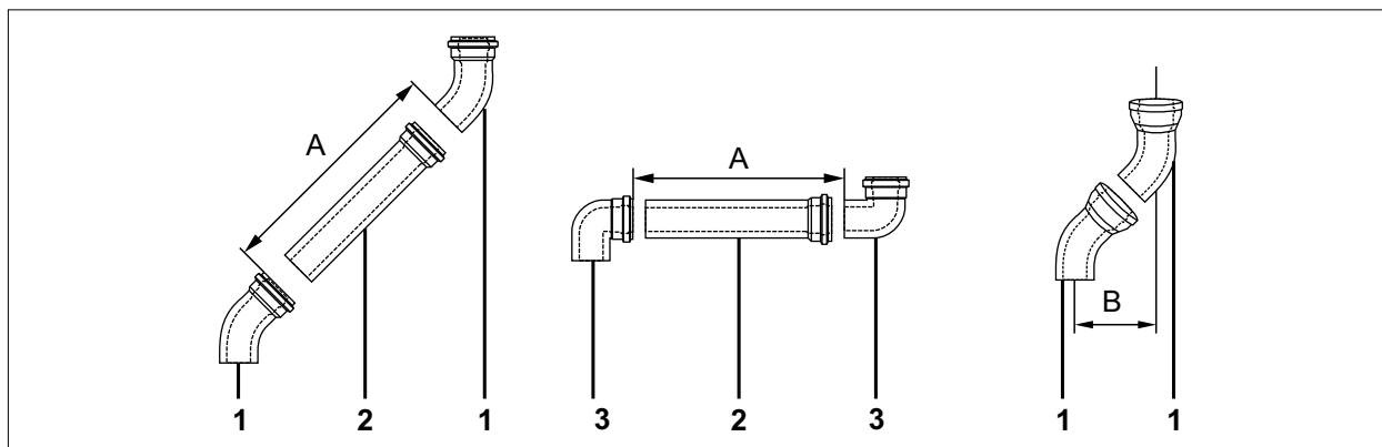
Abb. 5.14 Länge Luft-/Abgasrohr
