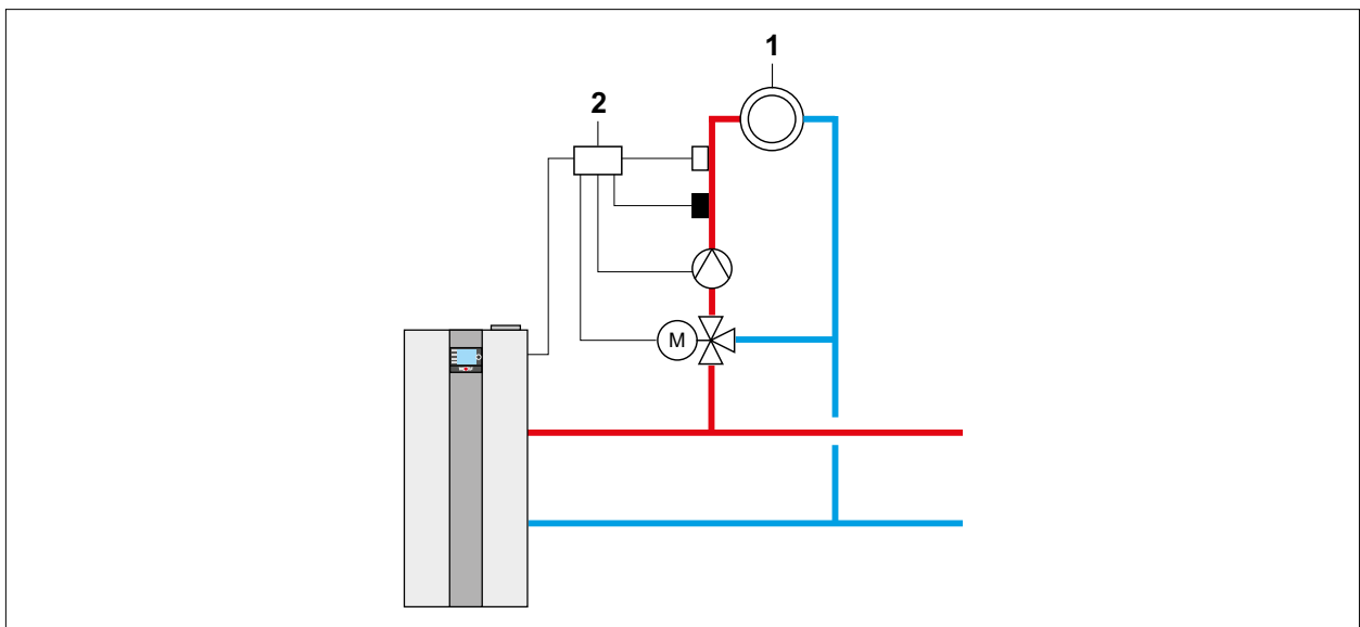
Abb. 13.5 Anlagenkonfiguration 02 - Ein oder mehrere Mischerkreise
