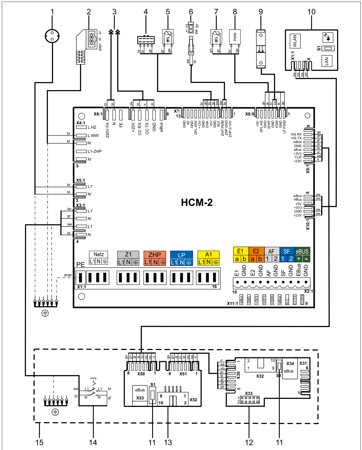
Abb. 13.1 Schaltplan HCM-2
