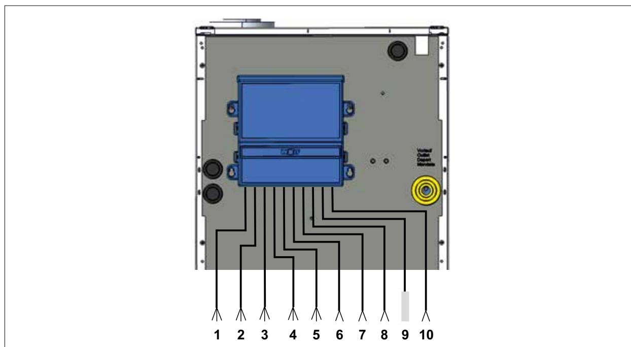
Abb. 5.23 Elektroanschluss Reglungskasten
