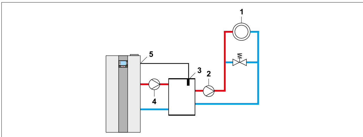
Abb. 13.9 Anlagenkonfiguration 12 - Hydraulische Weiche mit Sammlerfühler
