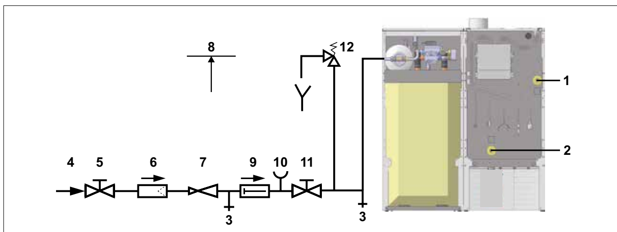
Abb. 5.9 Kaltwasseranschluss nach DIN 1988
