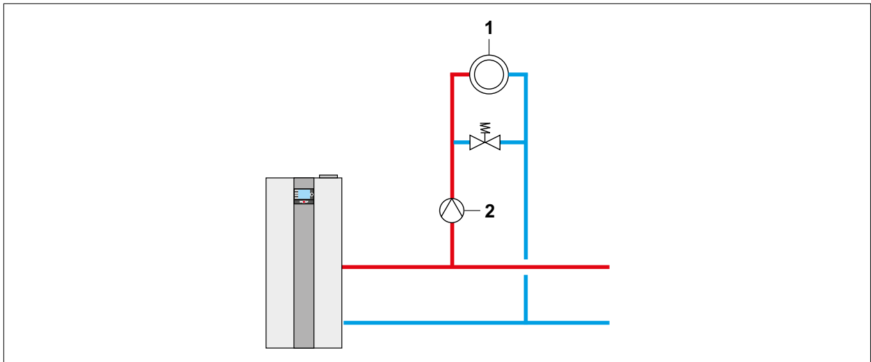
Abb. 13.4 Anlagenkonfiguration 01 - Direkter Heizkreis am Brennwertgerät + optional weitere Mischerkreise
