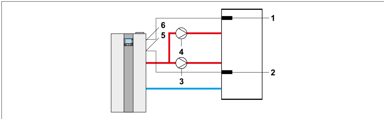
Abb. 13.8 Anlagenkonfiguration 11 - BSP-Speicher mit Sammlerfühler
