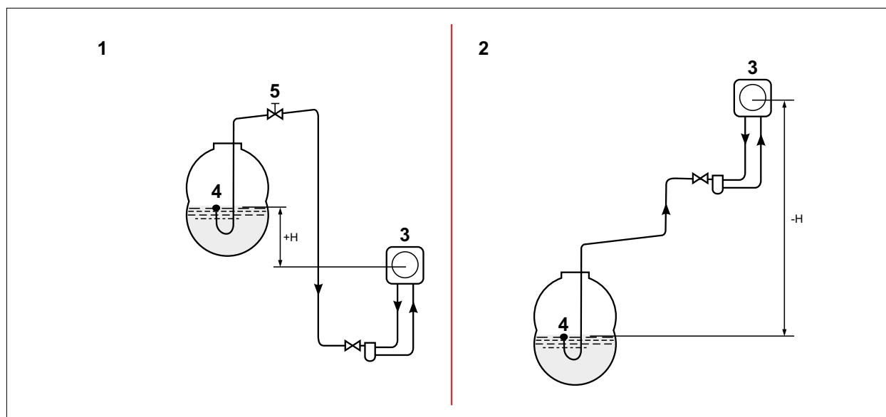
Abb. 4.3 Schwimmende Absaugung
