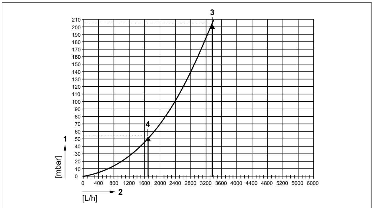
Abb. 12.8 Heizwasserseitiger Druckverlust COB-2-40
