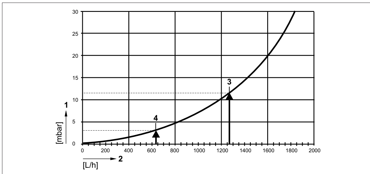
Abb. 12.5 Heizwasserseitiger Druckverlust COB-2-15
