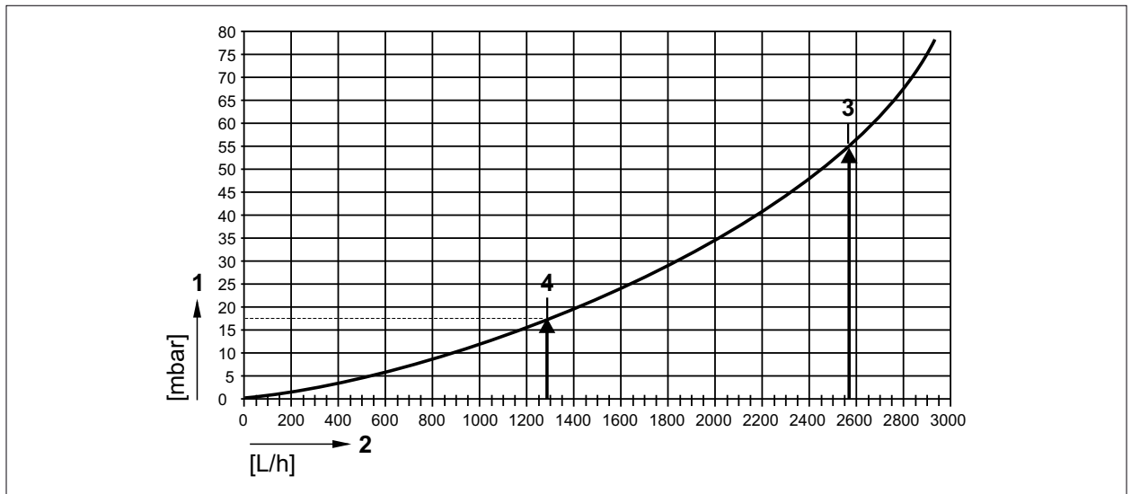
Abb. 12.7 Heizwasserseitiger Druckverlust COB-2-29
