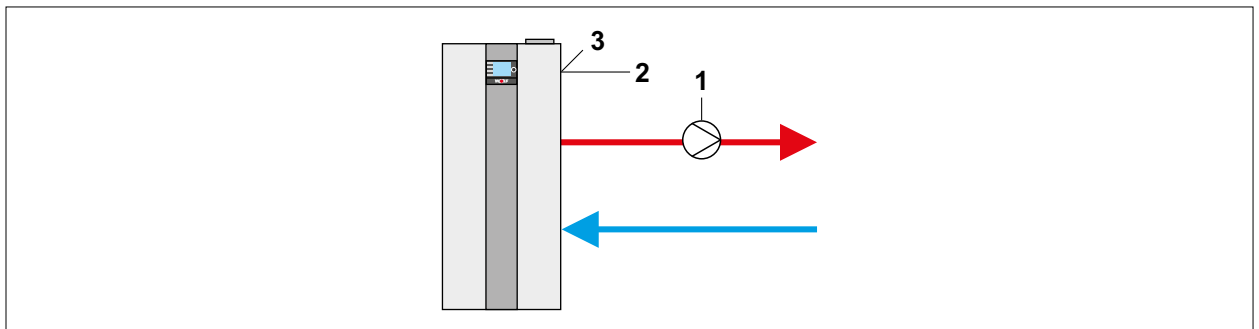
Abb. 13.11 Anlagenkonfiguration 52 - GLT - Kesselsolltemperatur
