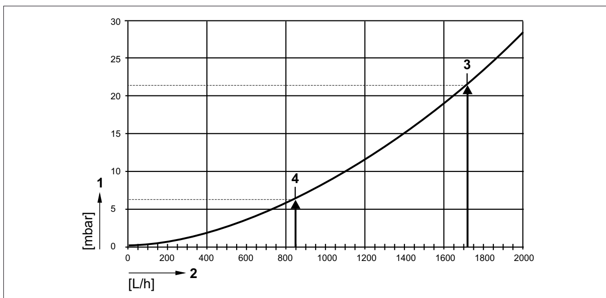
Abb. 12.6 Heizwasserseitiger Druckverlust COB-2-20
