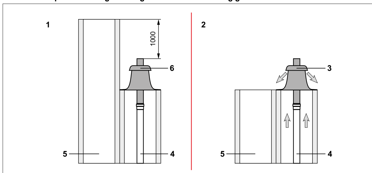
Abb. 4.6 Zweizügiger Schornstein
