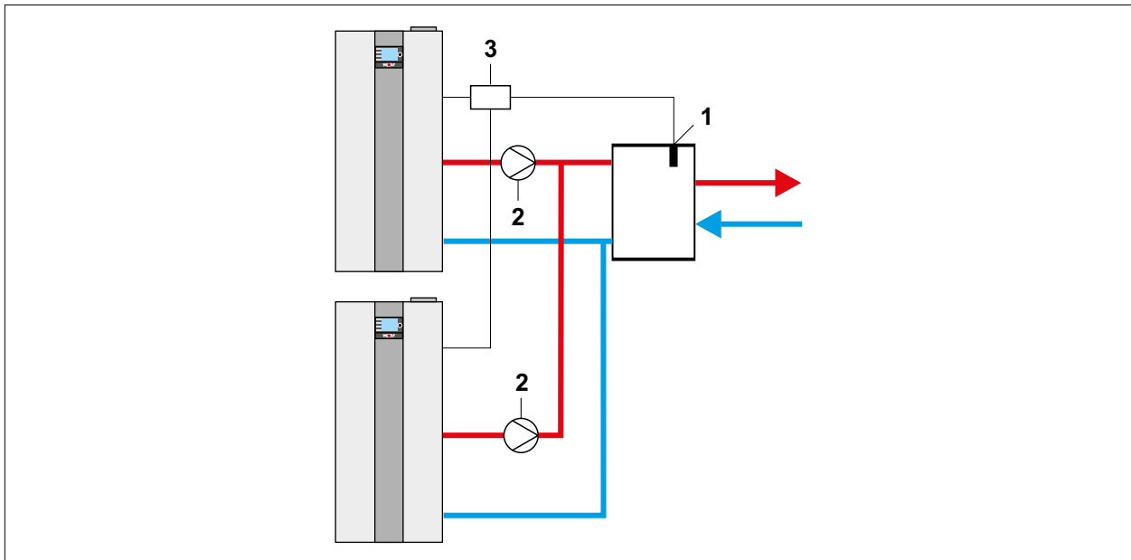
Abb. 13.12 Anlagenkonfiguration 60 - Kaskade für Mehrkesselanlagen
