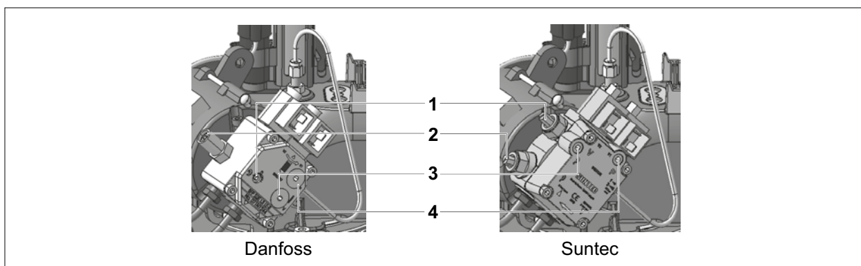
Abb. 6.6 Bauteile Ölpumpe
