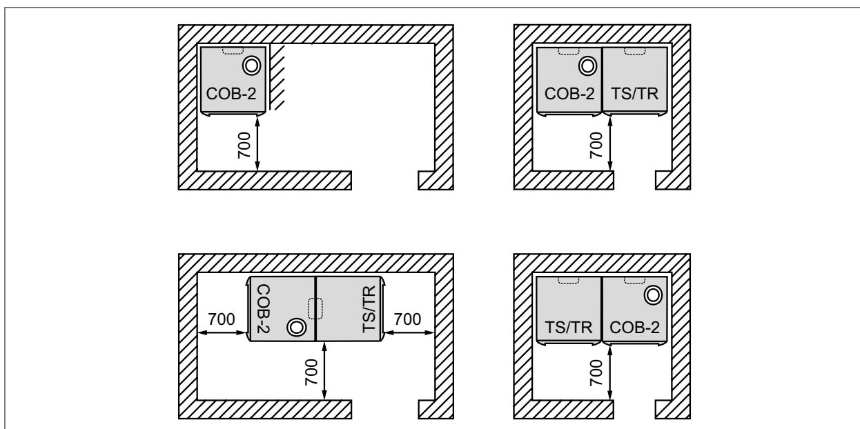
Abb. 4.1 Mindestwandabstände [mm]
