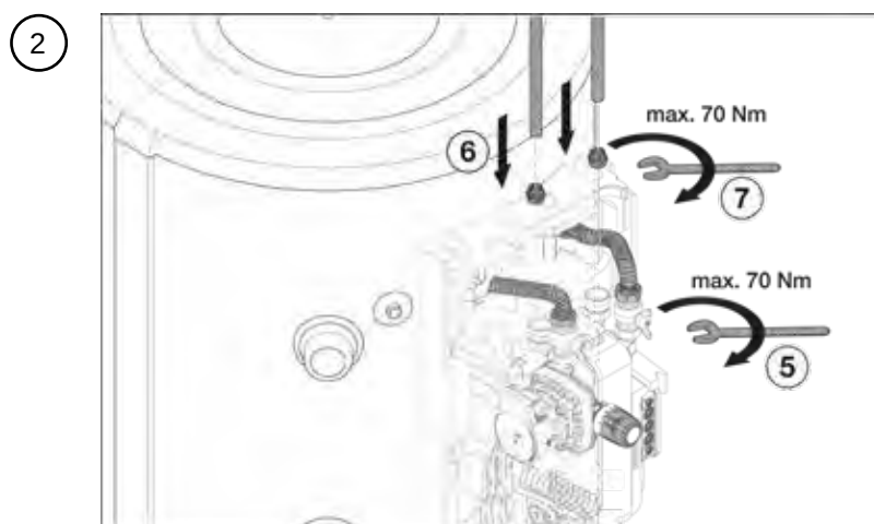
Montage des Anschlussets
