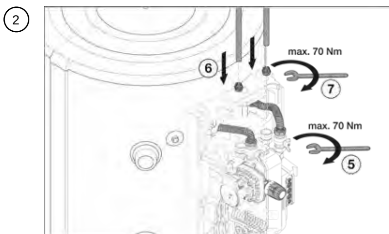
Montage du kit de raccordement
