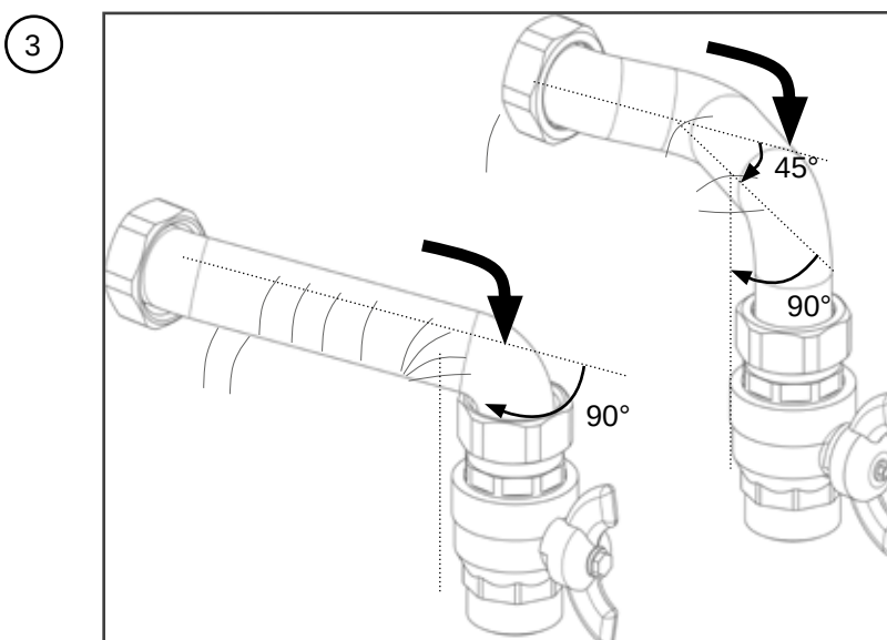
Formung des Anschlussets
