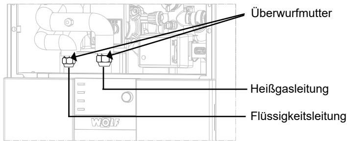
Abb.: Abb.: Kälteleitungen am Innenmodul anschließen
