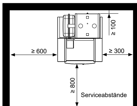
Draufsicht CHC-Split /200-35
