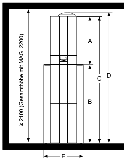
Vorderansicht CHC-Split /200
