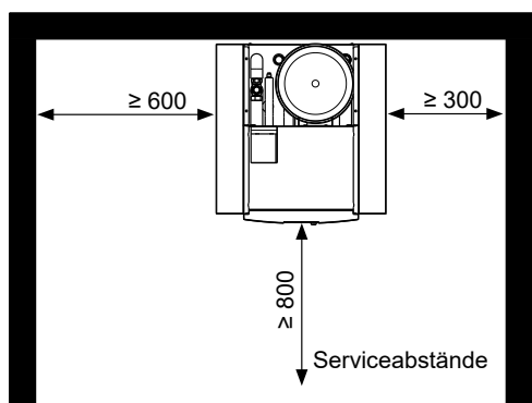
Draufsicht CHC-Split /200
