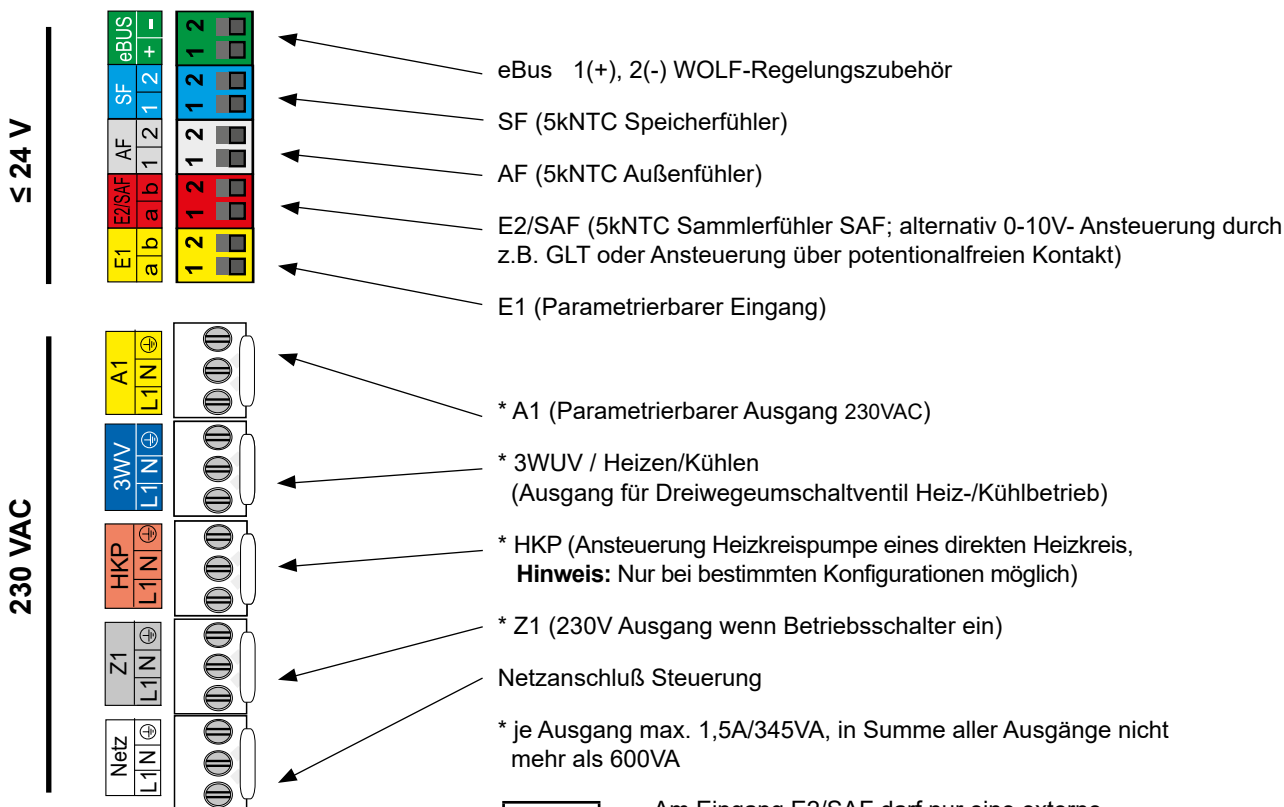
Bild: Regelungsplatine HCM-3
