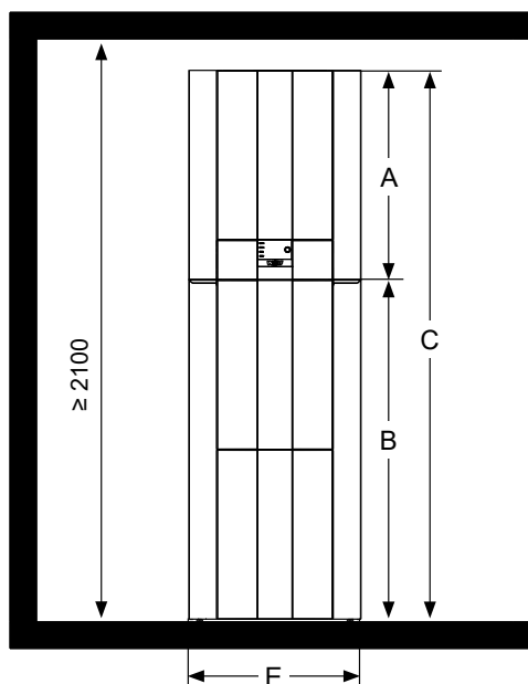
Vorderansicht CHC-Split /200-35
