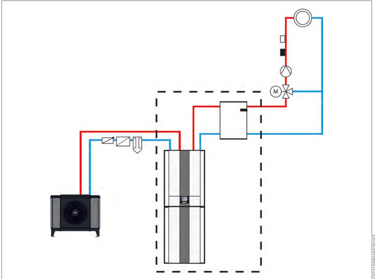
Wärmepumpencenter mit Trennspeicher und Mischerkreis
