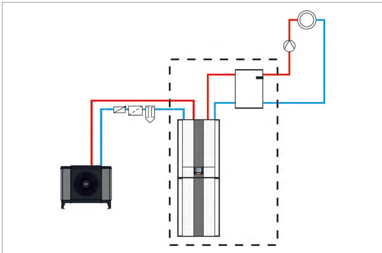
Wärmepumpencenter mit Trennspeicher und Heizkreis
