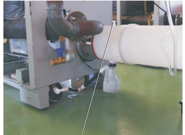
Messöffnung an der Kondensatfalle
