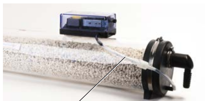
Luftschlauch
