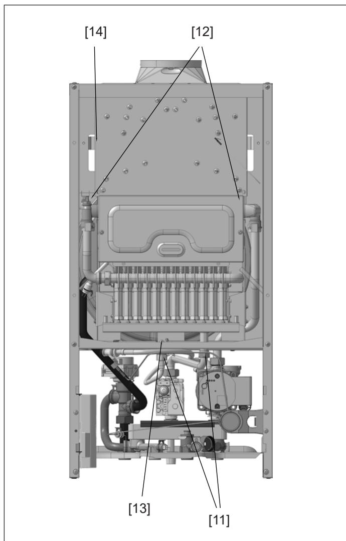
Bild: Tausch des Ausdehnungsgefäßes
