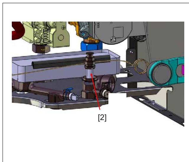
Bild: Kaltwassersieb
