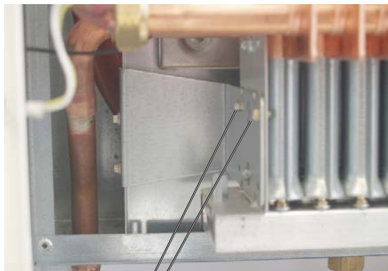
Befestigungsschrauben Brenneinheit [3] Achtung: parallel mit der anderen Seite durchführen
