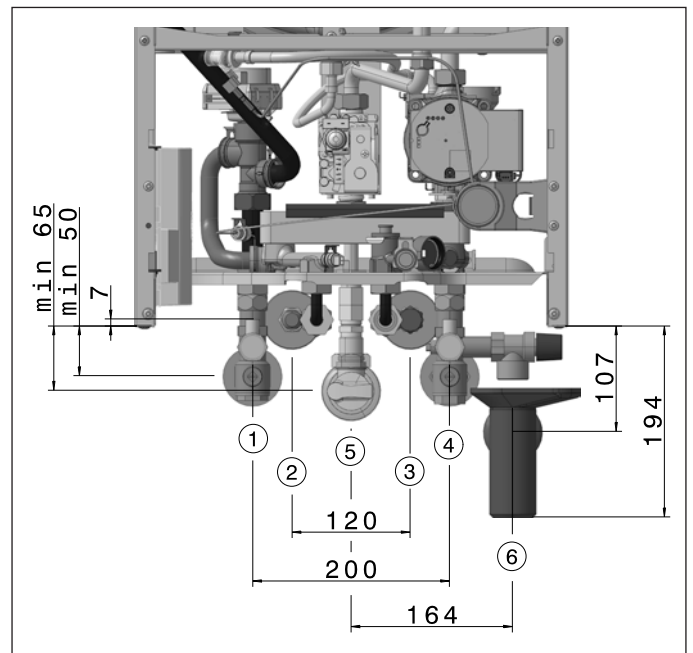
Bild: Vorderansicht Anschlussset für Unterputzinstallation
