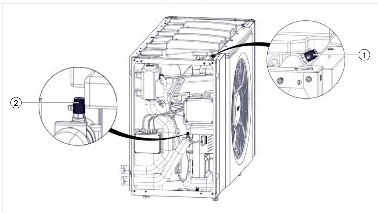
1 Handentlüfter (Luft-/Klätemittelabscheider)
