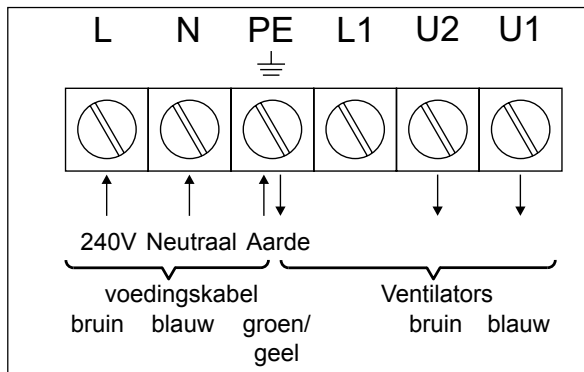
Aansluitschema
