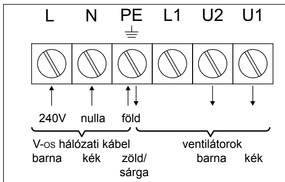
Anschlussbild
