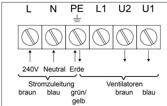
Anschlussbild
