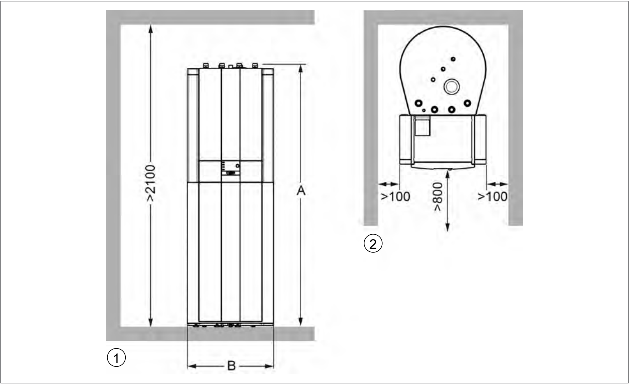
① Vorderansicht CHC-Monoblock / 300
