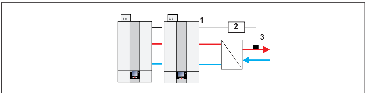
Abb. 14.9 Anlagenkonfiguration 60 - Kaskade für Mehrkesselanlagen
