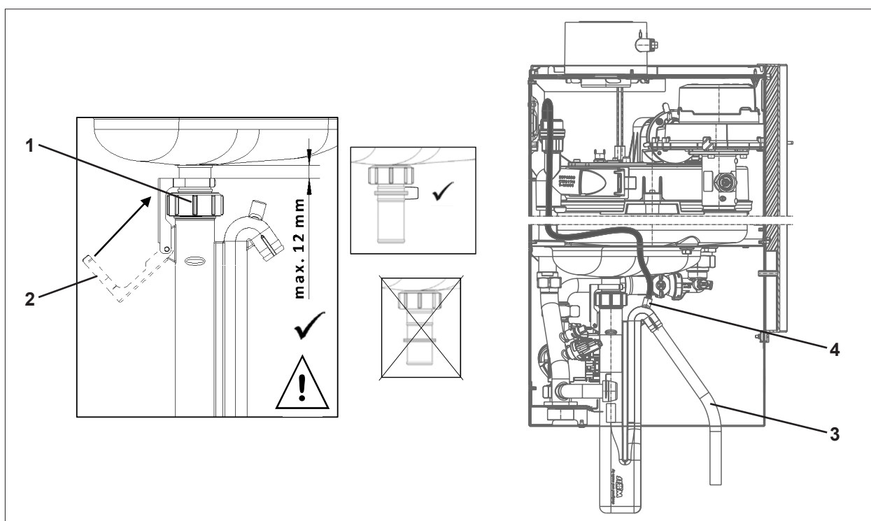
Abb. 5.6 Siphon
