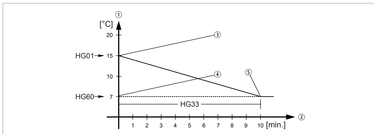
Abb. 7.1 Brennerhysterese
