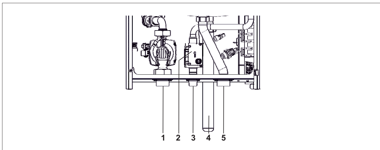
Abb. 13.2 Beschreibung Anschlüsse
