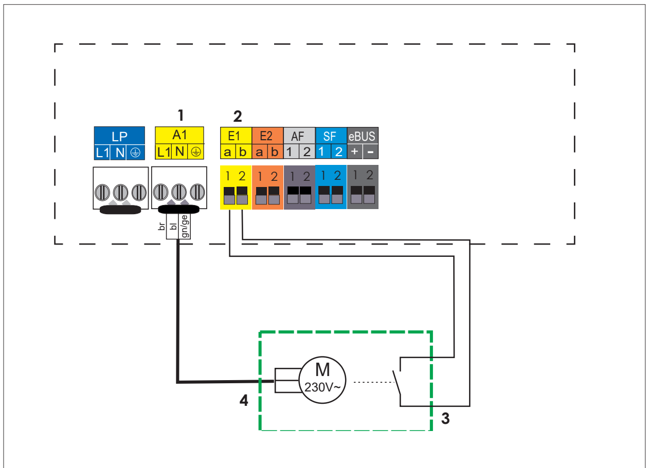
Abb. 5.25 Elektroanschluss Abgasklappe/Zuluftklappe
