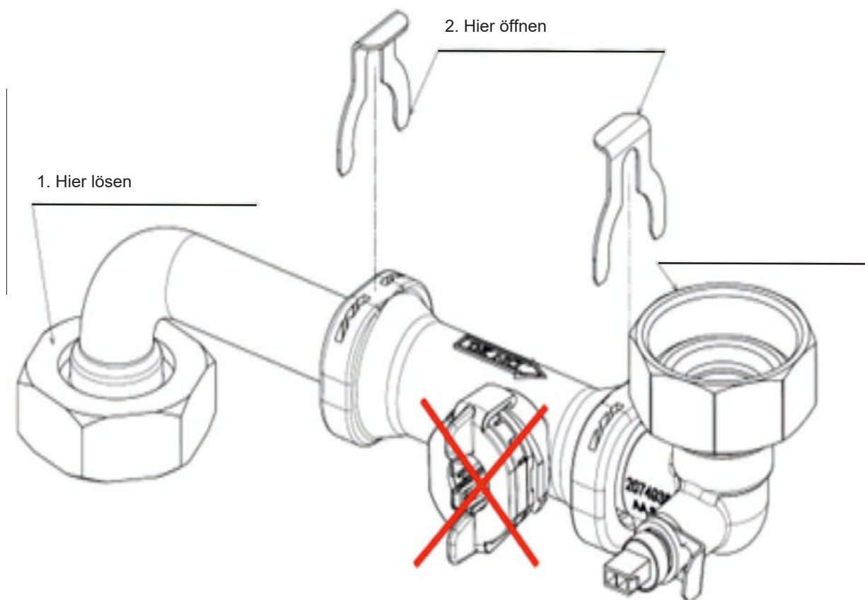
Abb. 10.2 Sensorelement wechseln
