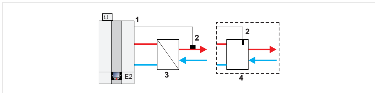
1 Eingang E2 3 Systemtrennung 2 Sammlerfühler 4 Hydraulische Weiche – Brenner geht nach Anforderung der Sammlertemperaturregelung in Betrieb. – Zubringer-/Heizkreispumpe als Zubringerpumpe aktiv. – Sammlertemperaturregelung – Eingang E2: Sammlerfühler – Parameter HG08 ( TV_{max} ): 90°C – Heizkreis (und Speicherladung) mit MM-2. – Speicherladung vor oder nach Hydraulischer Weiche; siehe 7.2.37 HG61: Warmwasser Regelung auf Seite 67
