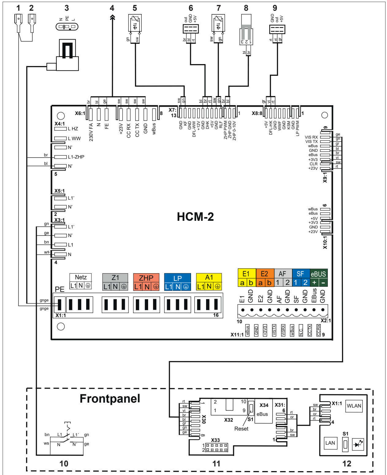
Abb. 14.1 Schaltplan HCM-2
