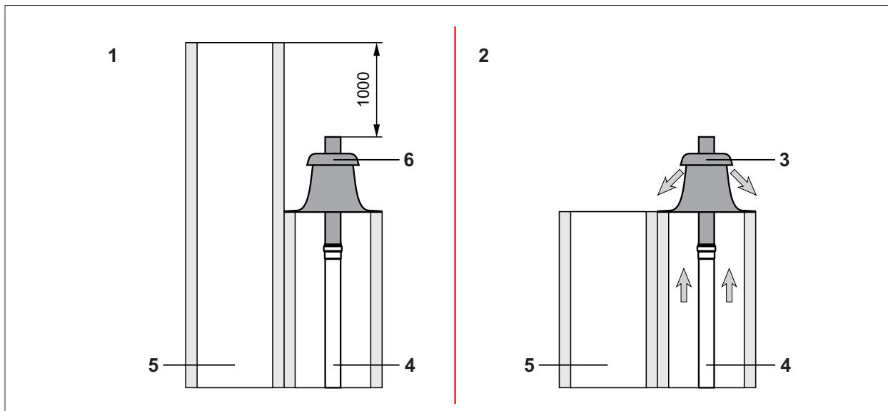
Abb. 4.12 Zweizügiger Schornstein
