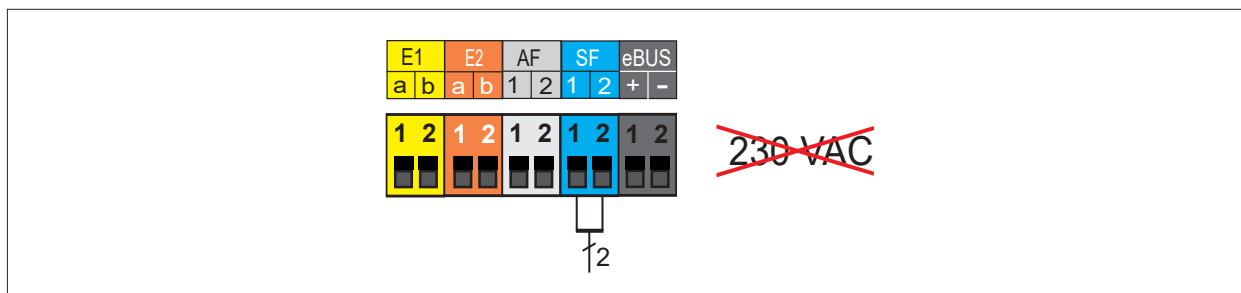
Abb. 5.23 Anschluss Speicherfühler
