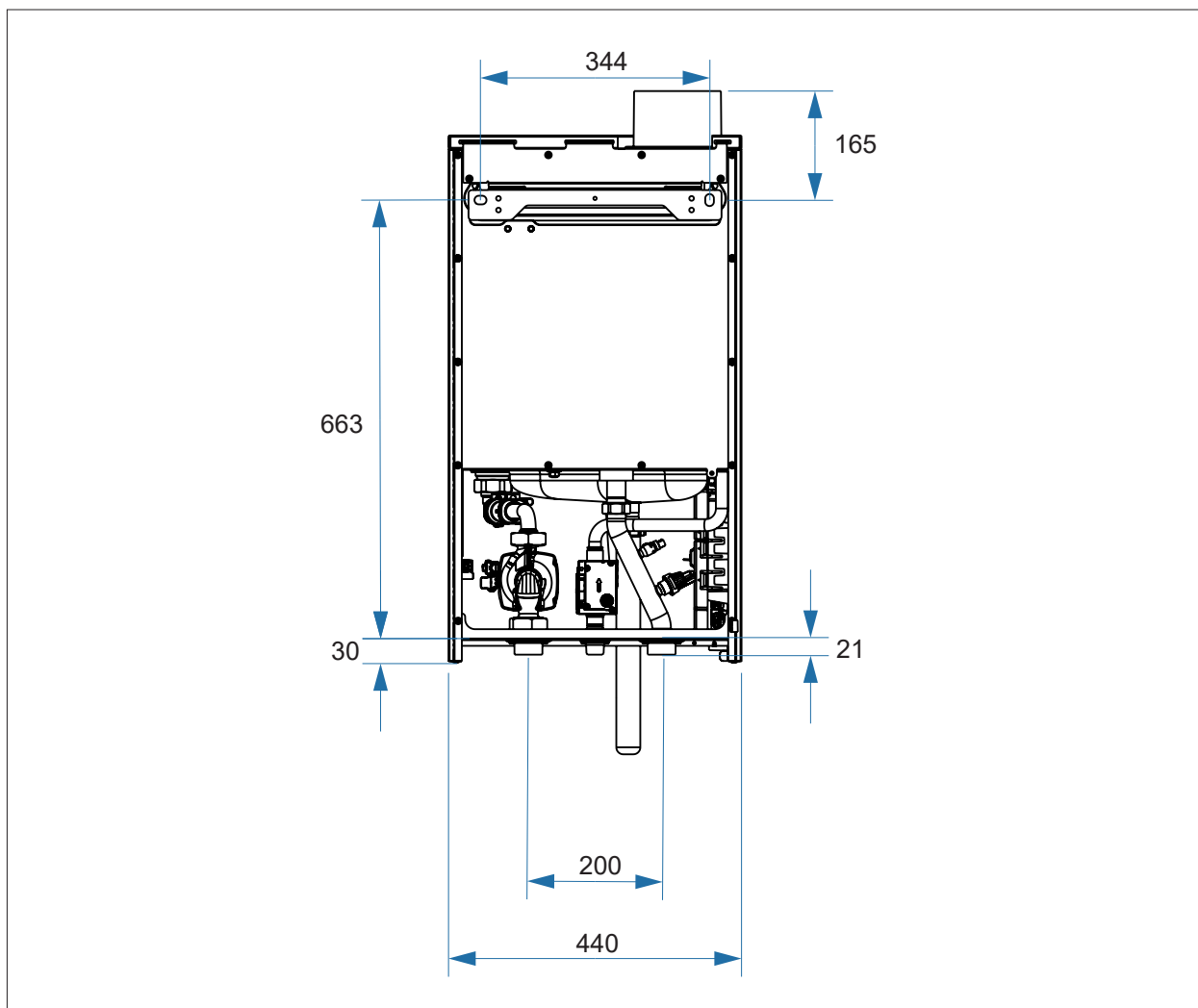
Abb. 13.1 Abmessungen Wärmerezeuger und Anschlüsse in mm
