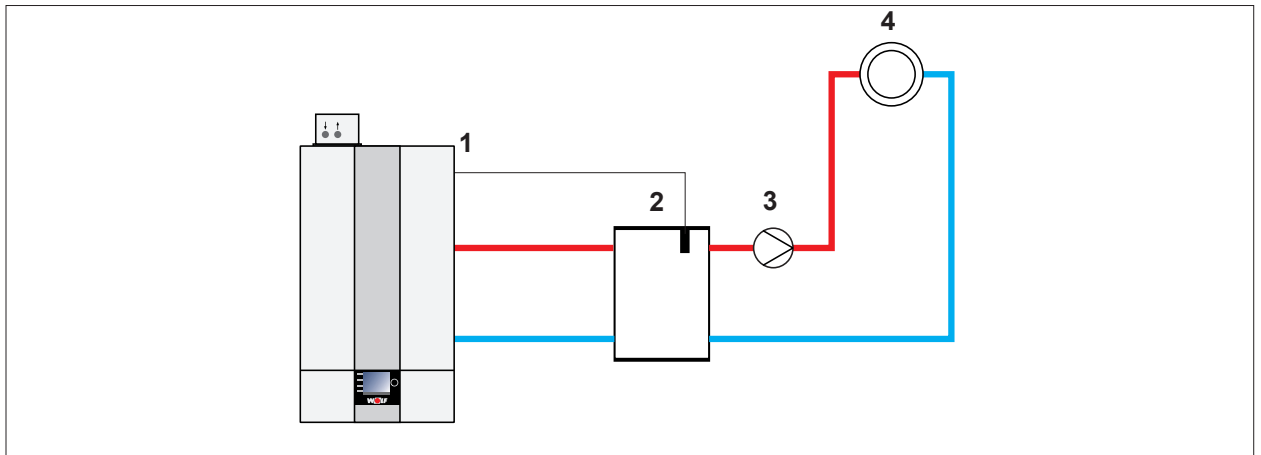
Abb. 14.6 Anlagenkonfiguration 12 - Hydraulische Weiche mit Sammlerfühler
