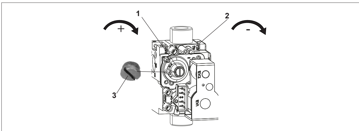
Abb. 6.3 Gaskombiventil
