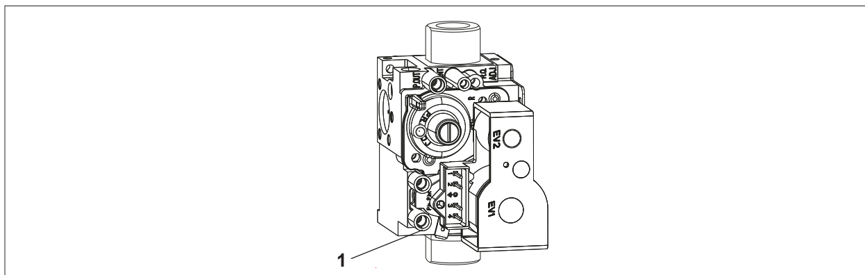
Abb. 6.1 Messnippel Gasdruck
