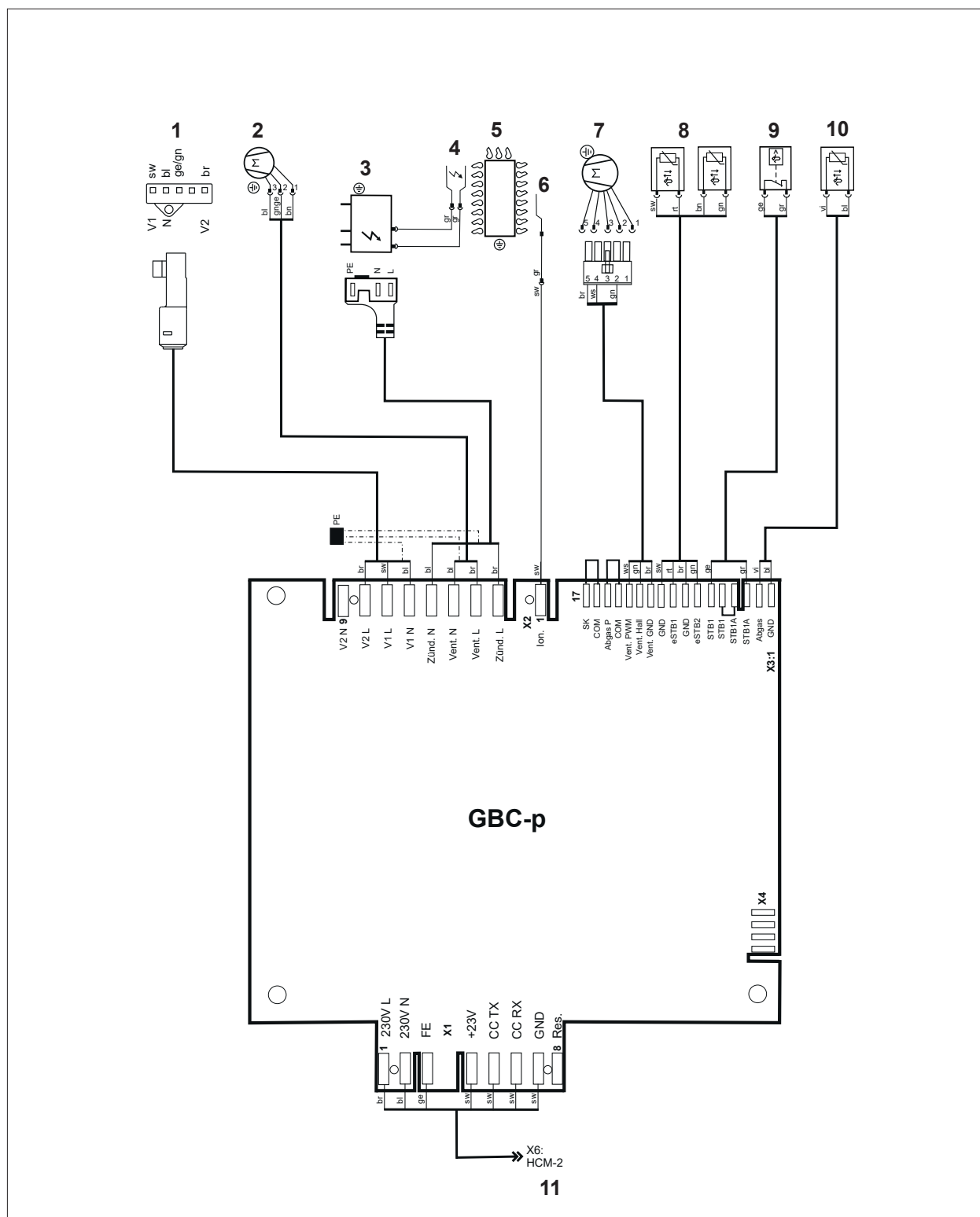
Abb. 14.2 Schaltplan GBC-p
