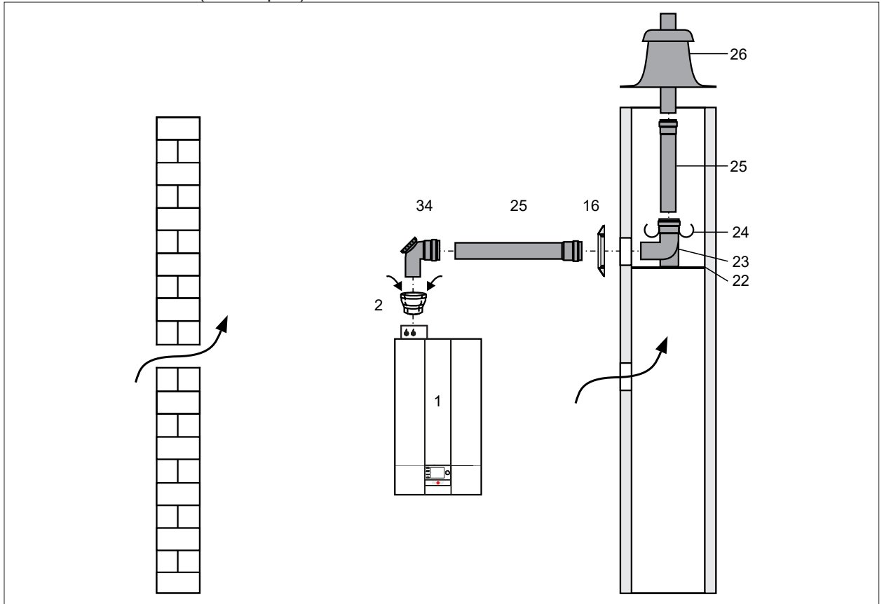
Abb. 4.10 Exzentrische Luft-/Abgasführung B23
