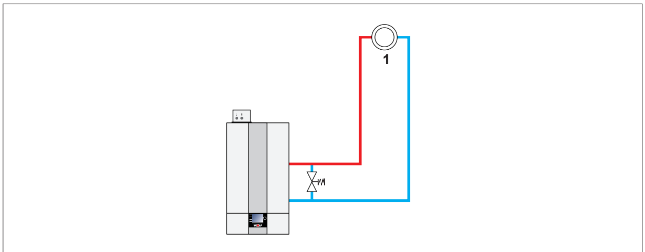
Abb. 14.3 Anlagenkonfiguration 01 - Direkter Heizkreis am Brennwertgerät + optional weitere Mischerkreise
