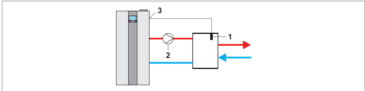
Abb. 14.6 Anlagenkonfiguration 11 - Hydraulische Weiche / Plattenwärmetauscher als Systemtrennung
