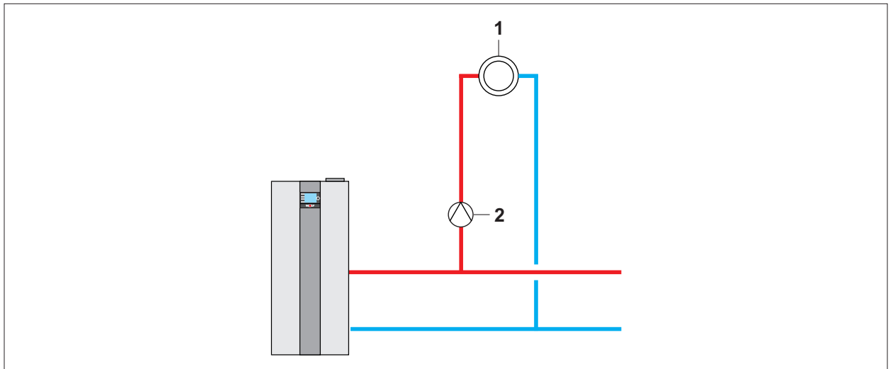
Abb. 14.4 Anlagenkonfiguration 01 - Direkter Heizkreis am Brennwertgerät + optional weitere Mischerkreise
