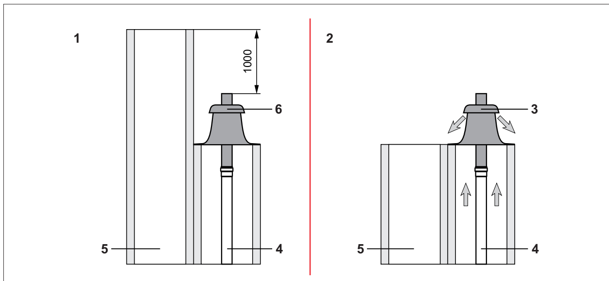
Abb. 4.13 Zweizügiger Schornstein
