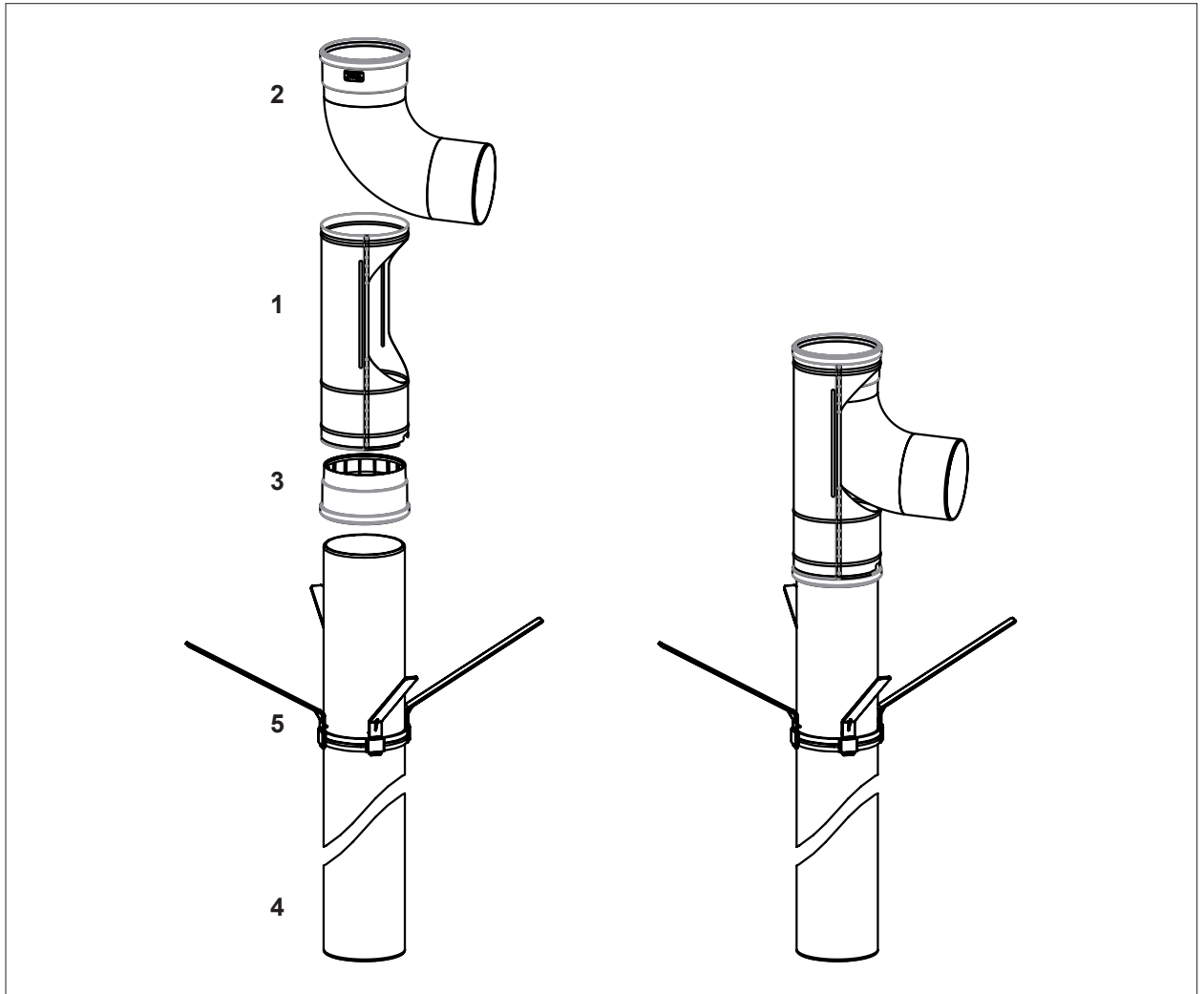
Abb. 4.12 Montage Stützrohr
