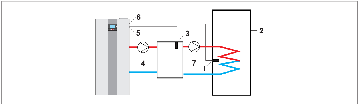
Abb. 14.8 Anlagenkonfiguration 11 - Speicher nach der Systemtrennung
