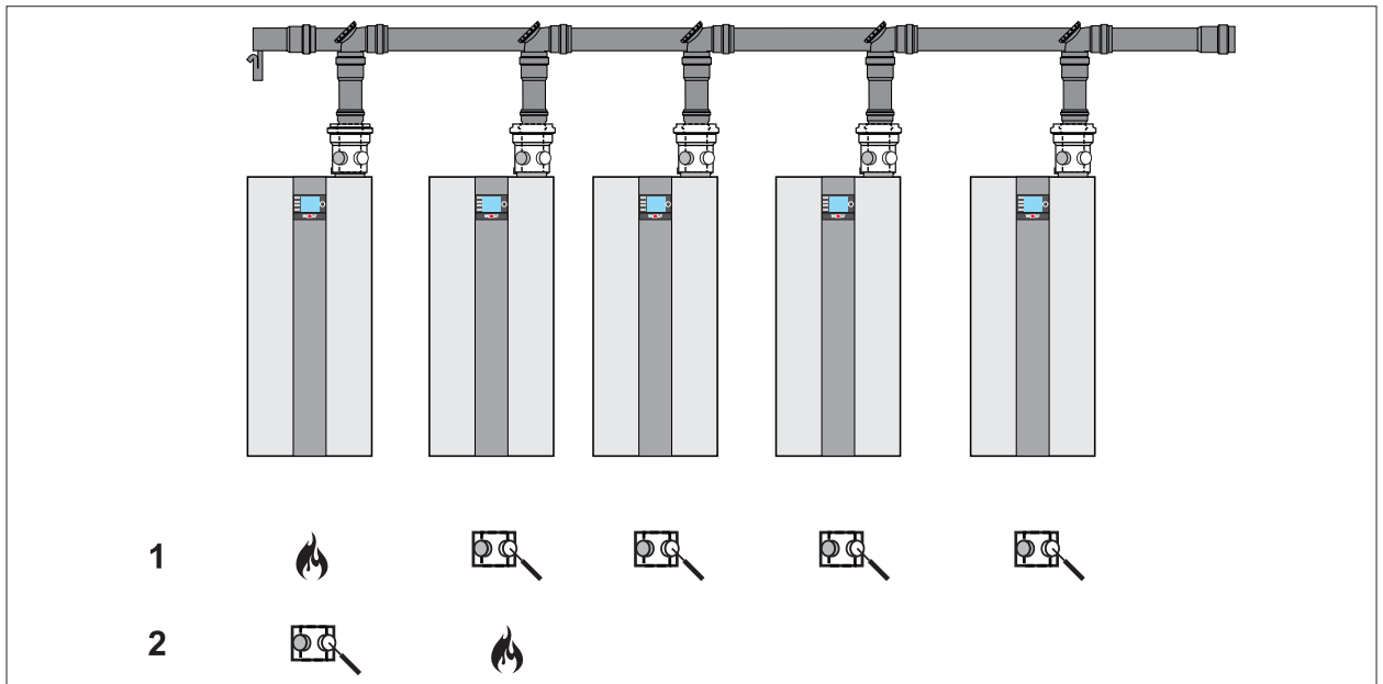
Abb. 6.7 Abgaskaskade
