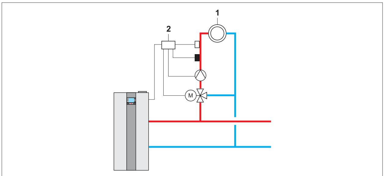
Abb. 14.5 Anlagenkonfiguration 02 - Ein oder mehrere Mischerkreise
