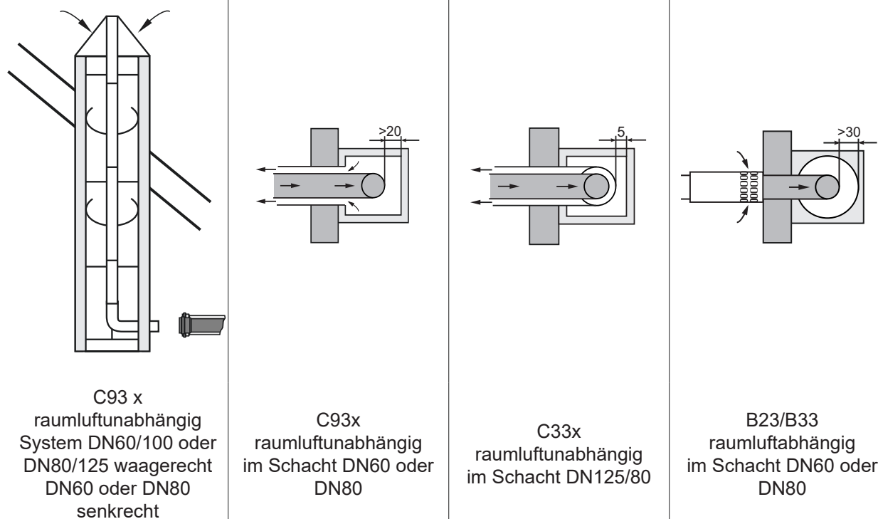
Abb. 4.5 Minimale Schachtgrößen
