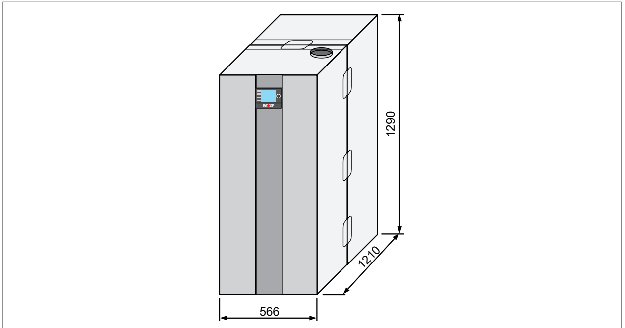
Abb. 13.3 Gasbrennwertkessel TGB-2 mit Speicher TS/TR, hinten stehend [mm]
