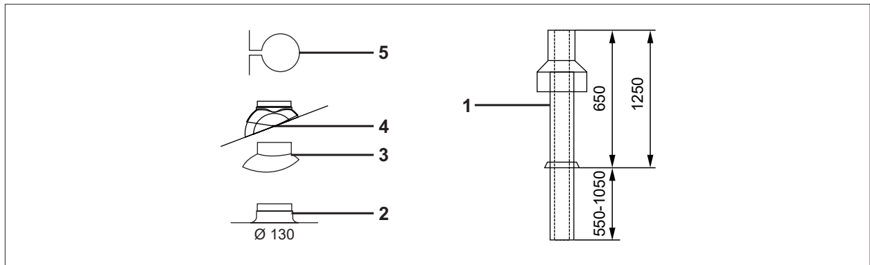
Abb. 5.18 Dachdurchführung [mm]
