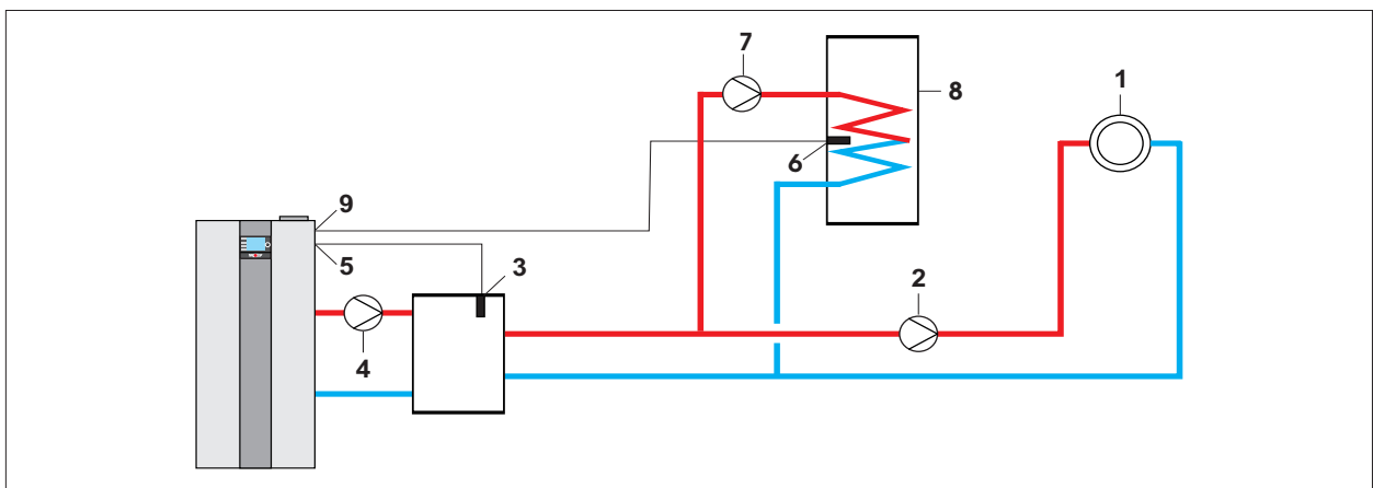
Abb. 14.11 Anlagenkonfiguration 12 - Hydraulische Weiche mit Sammlerfühler
