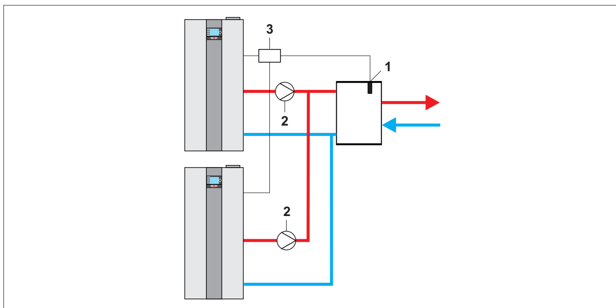
Abb. 14.14 Anlagenkonfiguration 60 - Kaskade für Mehrkesselanlagen
