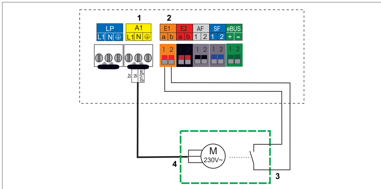
Abb. 14.3 Elektroanschluss Abgasklappe
