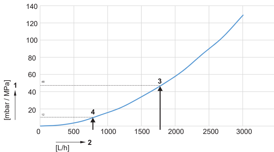
Abb. 13.5 Heizwasserseitiger Druckverlust TGB-2-20
