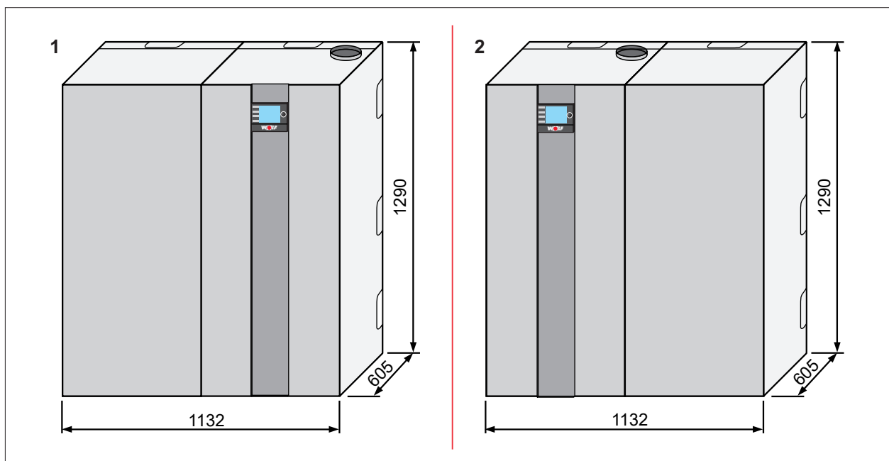
Abb. 13.2 Gasbrennwertkessel TGB-2 mit Speicher TS/TR
