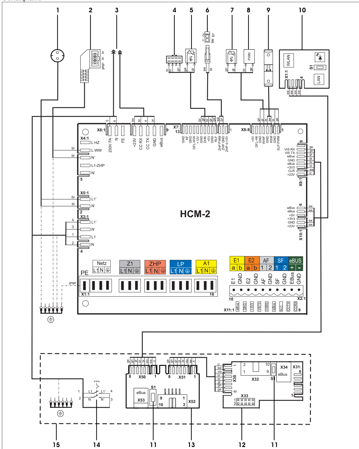
Abb. 14.1 Schaltplan HCM-2
