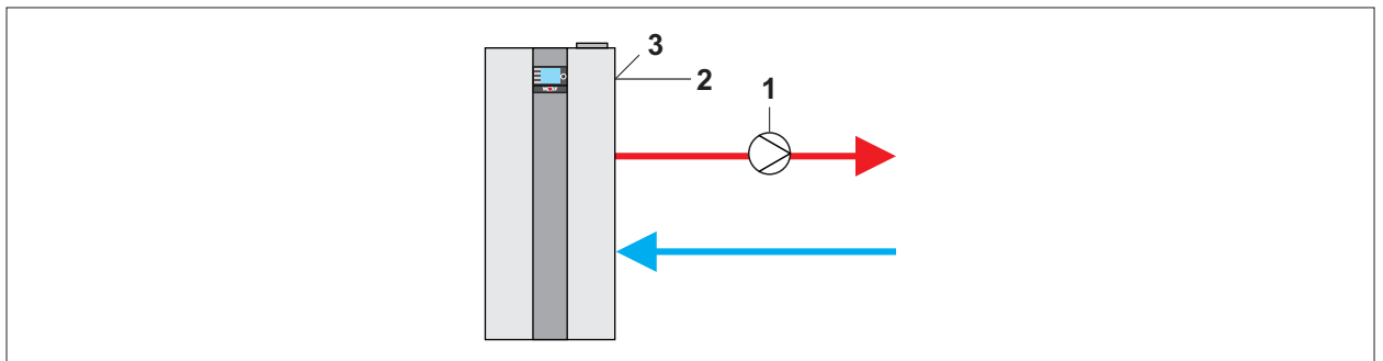
Abb. 14.13 Anlagenkonfiguration 52 - GLT - Kesselsolltemperatur
