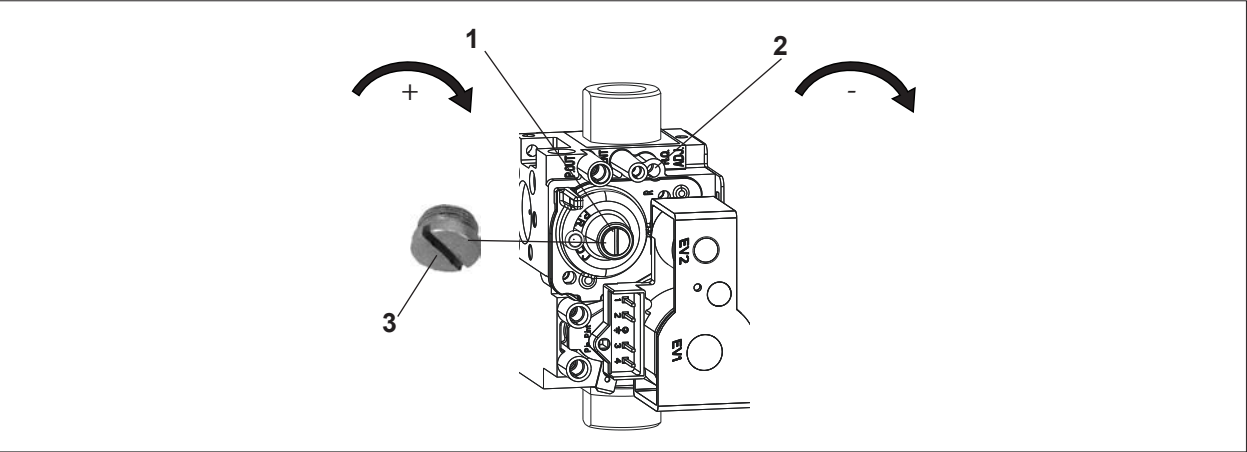
Abb. 6.6 Gaskombiventil 1 Nullpunktschraube (Untere Belastung) 3 Schutzschraube 2 Gasdurchflussschraube (Obere Belastung)
