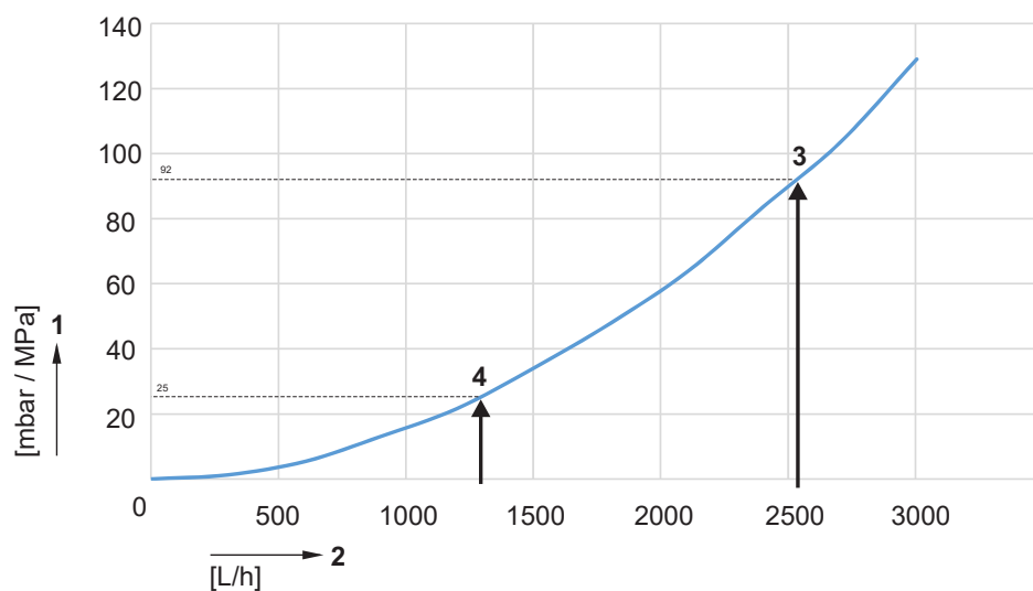
Abb. 13.6 Heizwasserseitiger Druckverlust TGB-2-30
