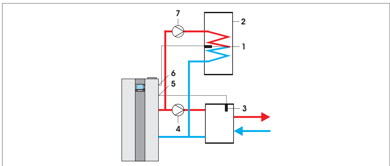
Abb. 14.7 Anlagenkonfiguration 11 - Speicher vor Systemtrennung
