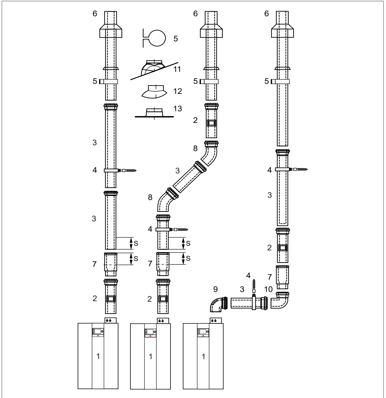
Abb. 4.6 Art C33x: Luft-/Abgasführung senkrecht über Dach.
