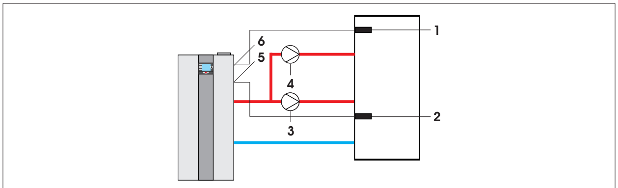
Abb. 14.9 Anlagenkonfiguration 11 - BSP-Speicher mit Sammlerfühler
