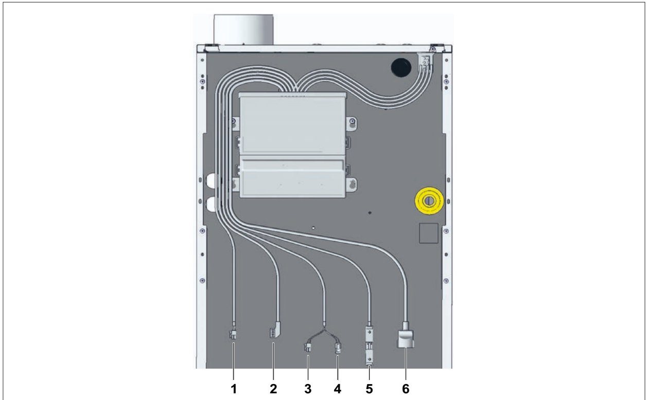
Abb. 5.22 Elektroanschluss des Anschlusskastens
