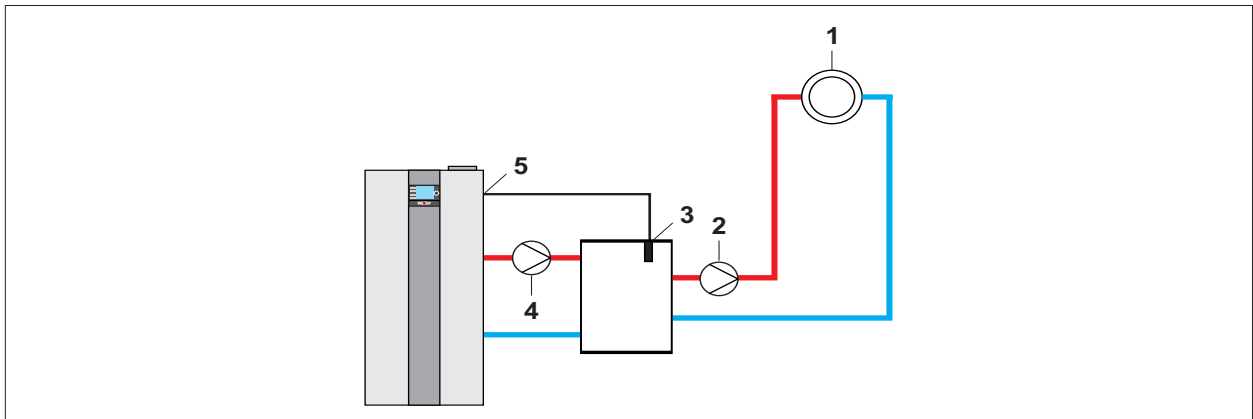
Abb. 14.10 Anlagenkonfiguration 12 - Hydraulische Weiche mit Sammlerfühler
