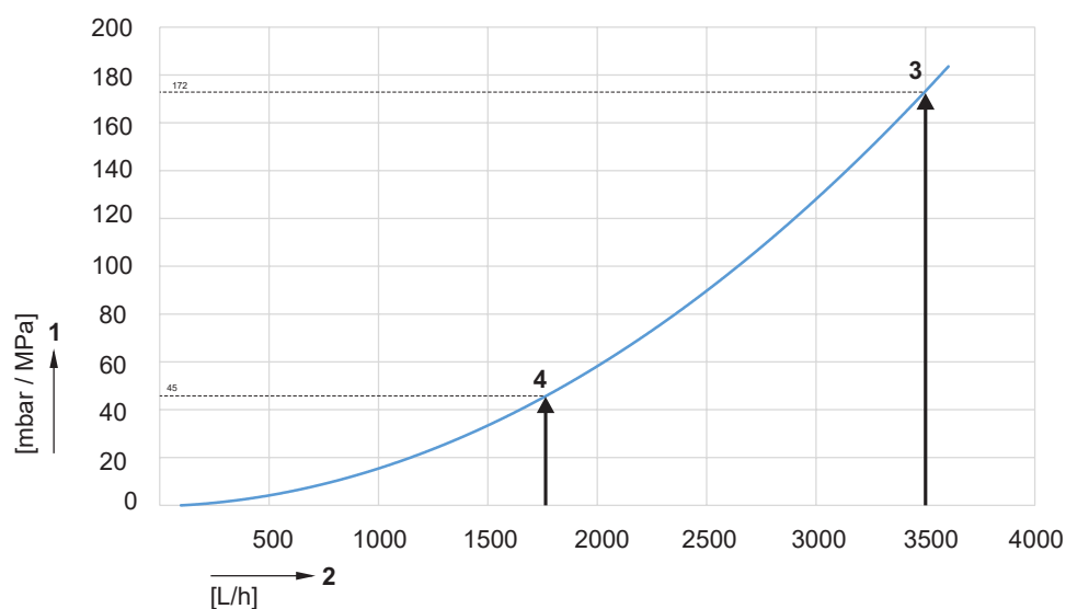
Abb. 13.7 Heizwasserseitiger Druckverlust TGB-2-40
