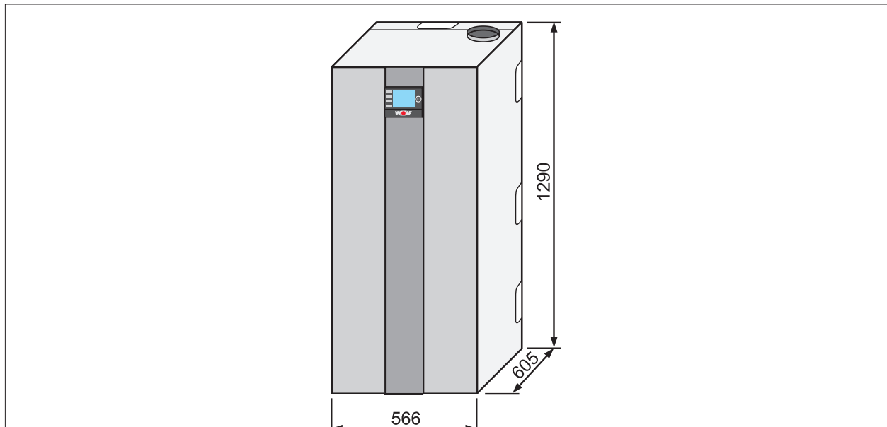
Abb. 13.1 Gasbrennwertkessel TGB-2 für Heizen mit Anschlussmöglichkeit für Speicherwassererwärmer z. B. SE-2, SEM-..., BSP [mm]
