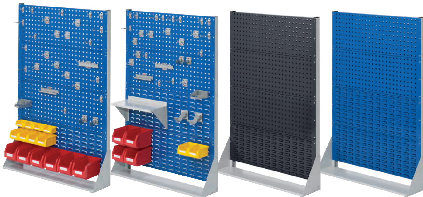
®RasterPlanStojany - Velikost 4 - V 1450 x Š 1000 x H 240 mm
