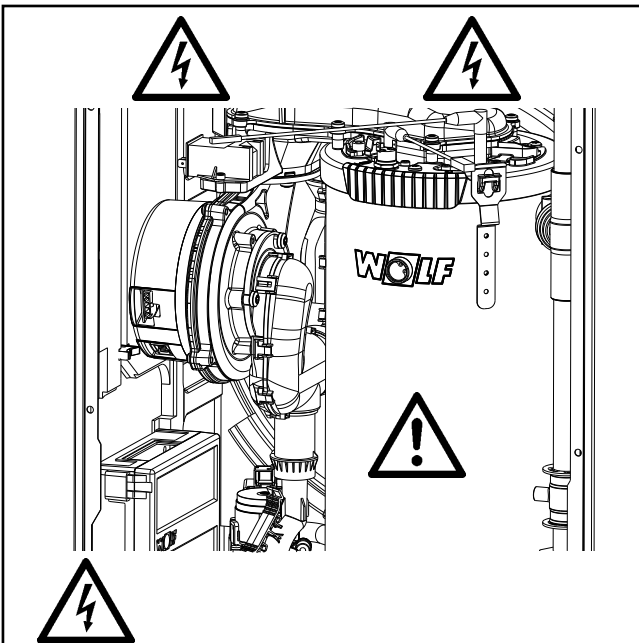
Bild: Zündtrafo, Hochspannung-Zünderlektrode, Brennkammer Gefahr durch elektrische Spannung, Gefahr von Verbrennung durch heiße Bauteile
