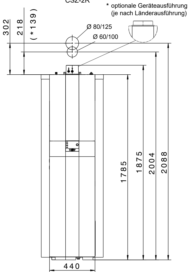
Vorderansicht CSZ-2R
