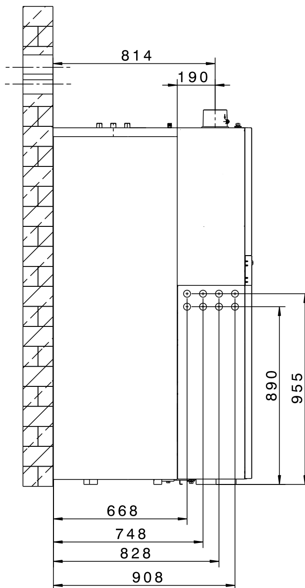
Seitenansicht CSZ-2R
