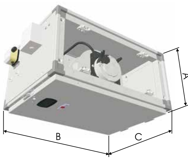
CFL-EC-ABL Abluftgerät
