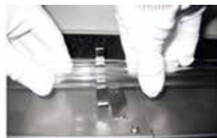
2. Įspauskite UVC fluorescencinį vamzdelį į priekinį laikiklį
