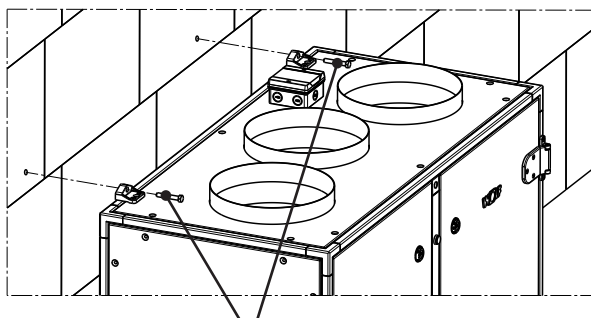
Befestigungsschrauben (bauseits)
