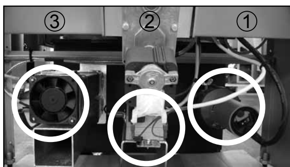
Abb. 26 von Links: Windrohr, Förderschneckenmotor, Zündgebläse
