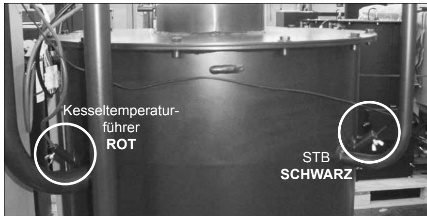
Abb. 32 Zwecks besserer Darstellung ohne Isolierung
