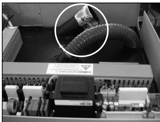
Abb. 07 Spannbrücke in montiertem Zustand mit Erdung (durch die sich im Förderschlauch befindende Erdungslitze).
