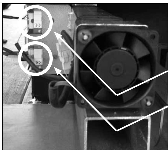
Abb. 27 Sekundär- und Primärwindrohr. Sensoren zeigen nach Außen!
