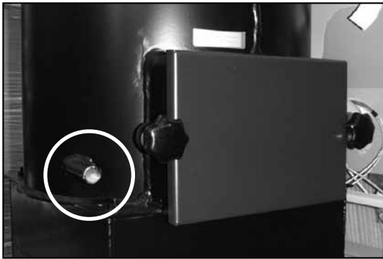
Abb. 08: Befüll- / Entleeranschluss BPH15, Anschluss 1/2 Zoll für KFE Hahn
