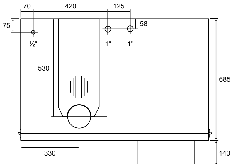
Abb. 09 Abmessungen Anschlüsse
