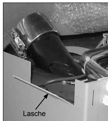
Abb. 43 Nach außen gebogene Lasche, Durchführung für Zuleitungen (Pumpen etc.)
