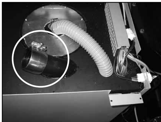
Abb. 07 Spannbrücke in montiertem Zustand mit Erdung (durch die sich im Förderschlauch befindende Erdungslitze).
