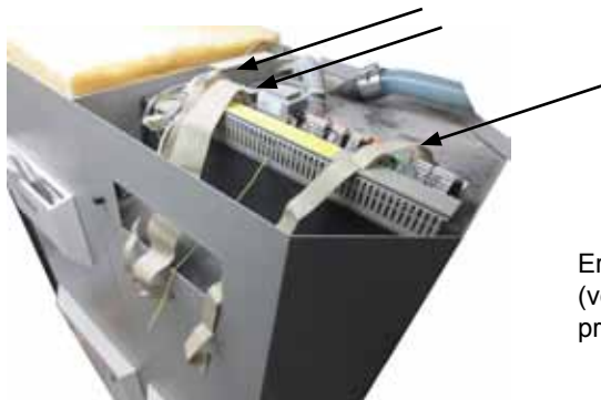
Abb. 47.1 Anschluss Flachkabel an Hauptklemmenprint
