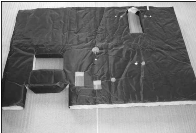
Abb. 02: Wickelisolierung
