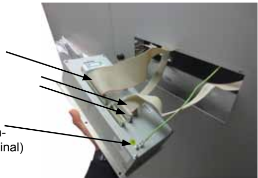
Abb. 47.2 Anschluss Flachkabel an Terminal
