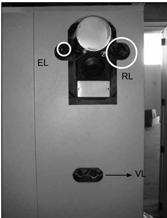
Abb. 10 BPH25/BPH35: Rücklauf / Vorlauf / Entlüftung (Bei 35kW entspricht das Saugzuggebläse nicht der Abb.)
