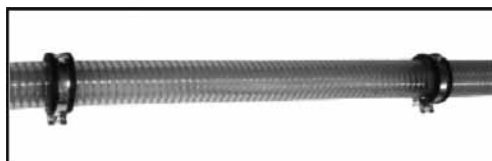
Abb.: Pelletsschlauch. Nicht quetschen. Erdung nicht vergessen.
