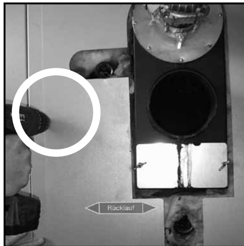
Abb. 53 Befestigung der Rauchkastenabdeckung (Rückseite) mittels Akku-Schrauber & mitgelie- ferter Schraube.
