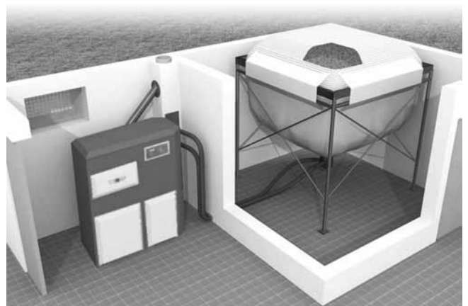
Sacksilo
