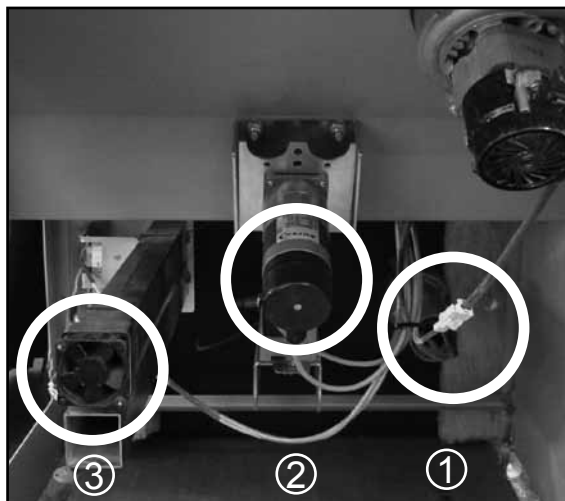
Abb. 25 von Links: Windrohr, Förderschneckenmotor, Zündgebläse
