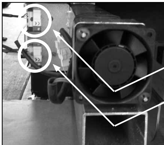
Abb. 26 Sekundär- und Primärwindrohr. Sensoren zeigen nach Außen!
