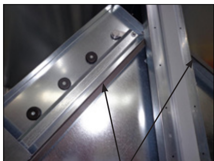
Étanchéifier sur toute la circonférence
