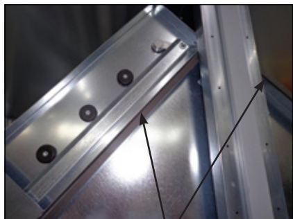
Герметизировать по периметру
