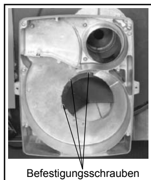
Bild: Ansaugluftführung (ALF)
