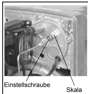
Bild: Düsenstockeinstellung
