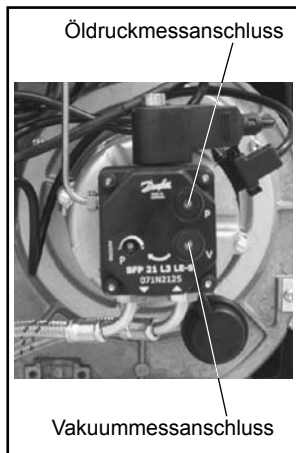
Bild: Unterdruckkontrolle
