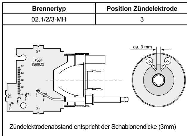
Bild: Einstellung Zündelectroden
