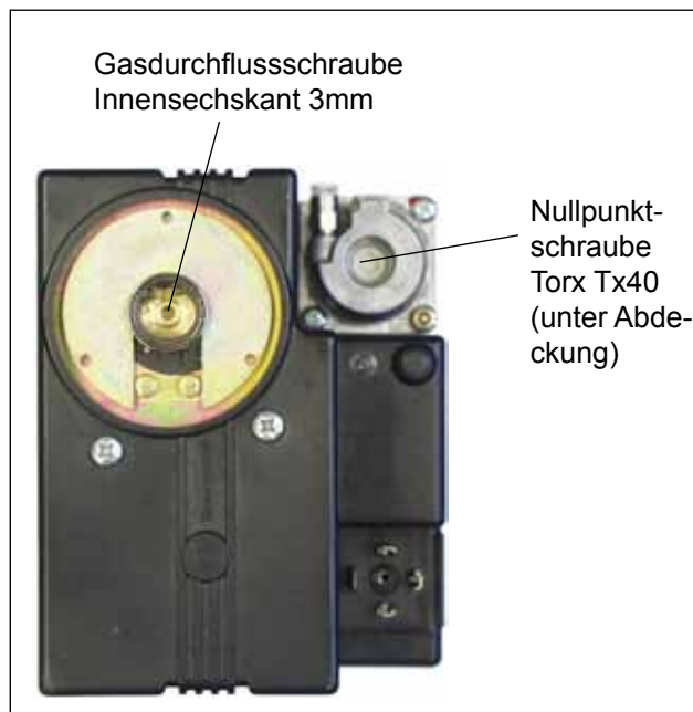
Bild: Gaskombiventil
