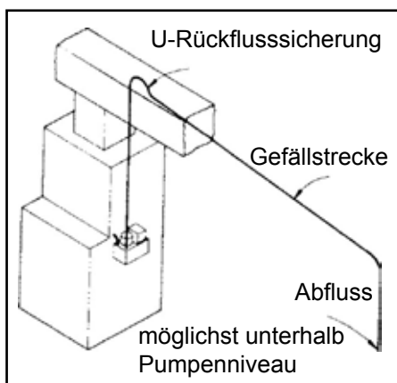
Anschluss an den Abfluss
