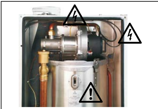
Bild: Zündtrafo, Hochspannungs-Zündeletrode, Wärmetauscher Gefahr durch elektrische Spannung, Gefahr von Verbrennung durch heiße Bauteile
