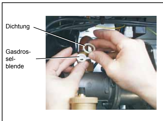
Bild 3: Gasdrosselblende mit Dichtung einsetzen
