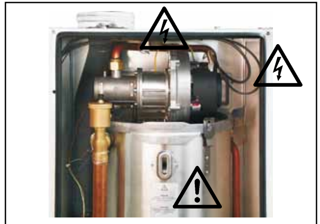
Bild: Zündtrafo, Hochspannungs-Zündelectrode, Wärmetauscher
