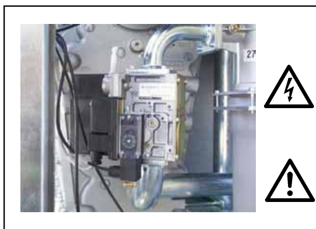
Bild: Gaskombiventil MGK-170/210/250/300 Gefahr durch elektrische Spannung Gefahr von Vergiftung und Explosion durch ausströmendes Gas
