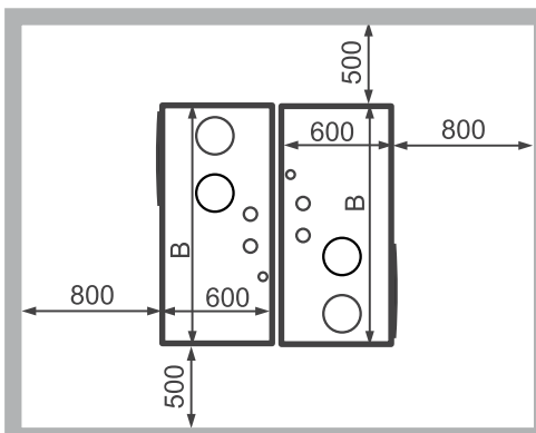
2 Kessel im Heizraum, Rückseite aneinander
