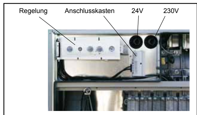
Bild: Regelung MGK-170/210/250/300
