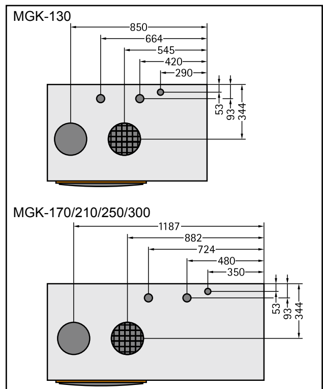
Bild: Anschlussmaße
