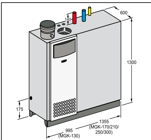
Bild: Abmessungen (Gesamthöhe inkl. Anschlussstutzen MGK-130 ... 250 = 1460 mm MGK-300 = 1510 mm)
