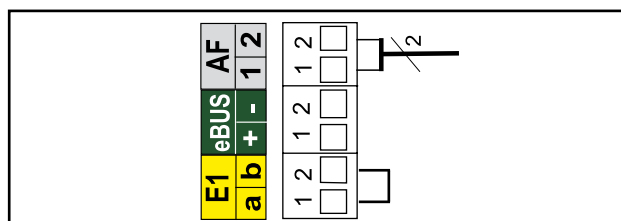
Bild: Anschluss Außenfühler
