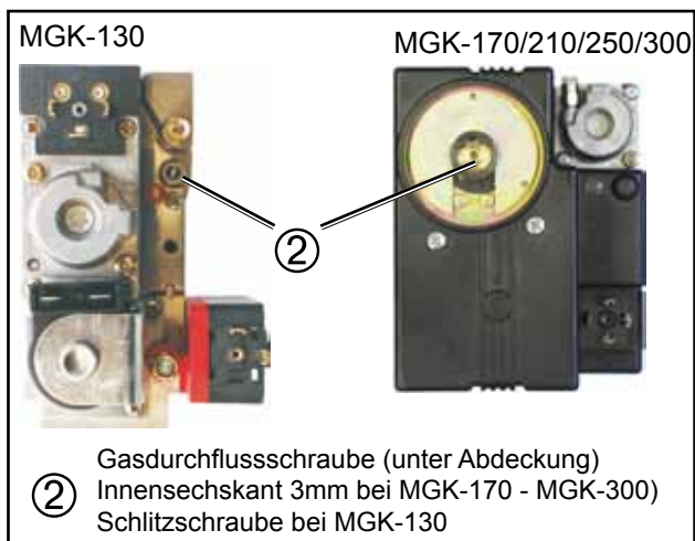
Bild: Gaskombiventil
