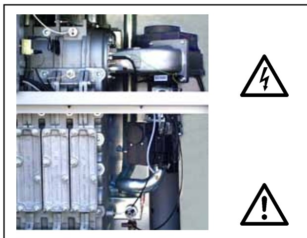
Bild: Zündtrafo, Hochspannungs-Zünderlektrode, Brennkammer Gefahr durch elektrische Spannung, Gefahr von Verbrennung durch heiße Bauteile
