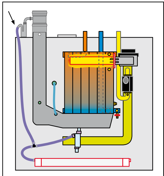
Bild: Kondensatschlauch
