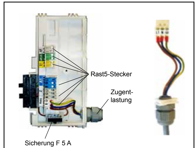
Bild: Anschlusskasten
