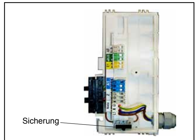
Bild: Anschlusskasten-Abdeckung geöffnet
