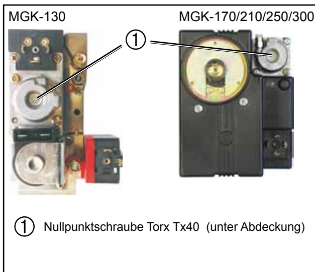
Bild: Gaskombiventil
