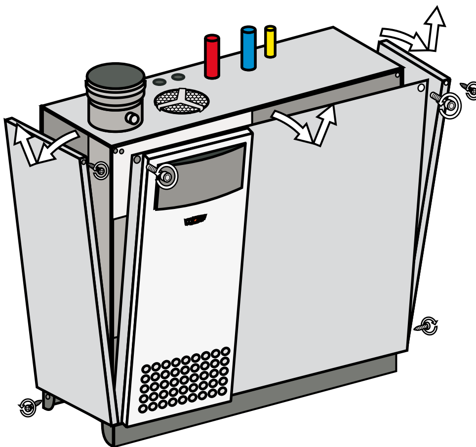
Bild: Demontage der Frontverkleidung und der Seitenverkleidung
