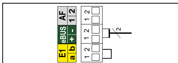
Bild: Anschluss Wolf-Regelungszubehör digital (eBus-Schnittstelle)
