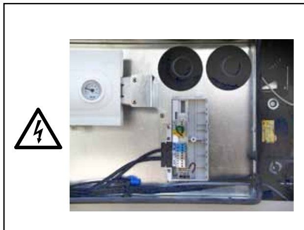
Bild: Anschlusskasten MGK-170/210/250/300 Gefahr durch elektrische Spannung
