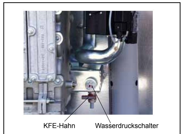
Bild: KFE-Hahn
