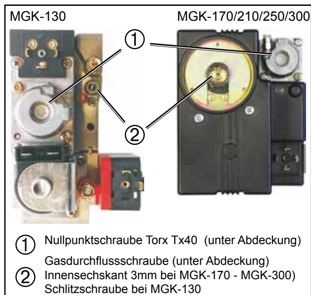
Bild: Gaskombiventil
