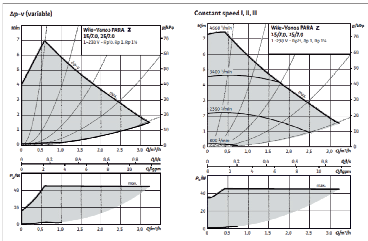
Abb. 6.3 Kennlinien Zirkulationspumpe
