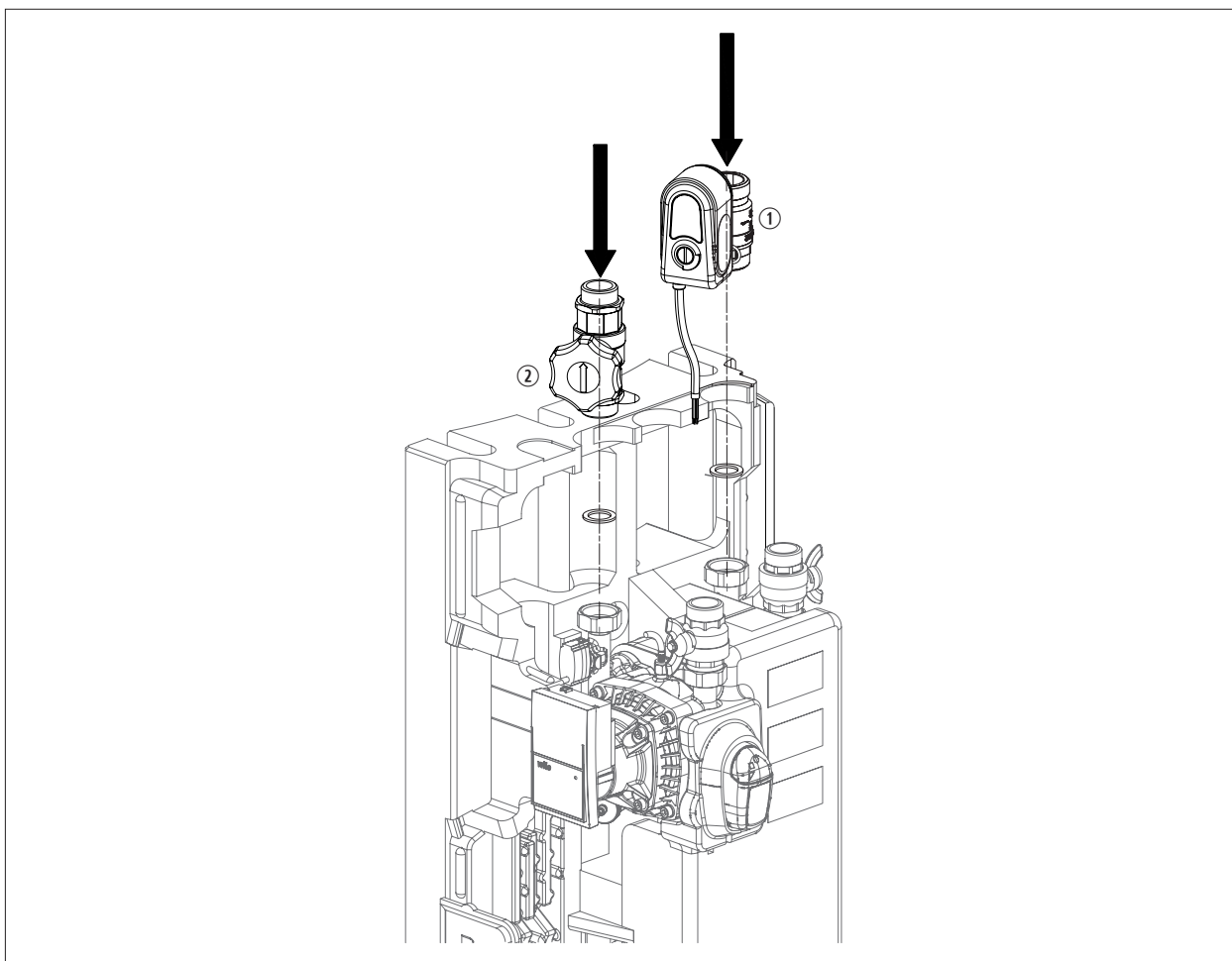
Abb. 3.6 Zubehör montieren
