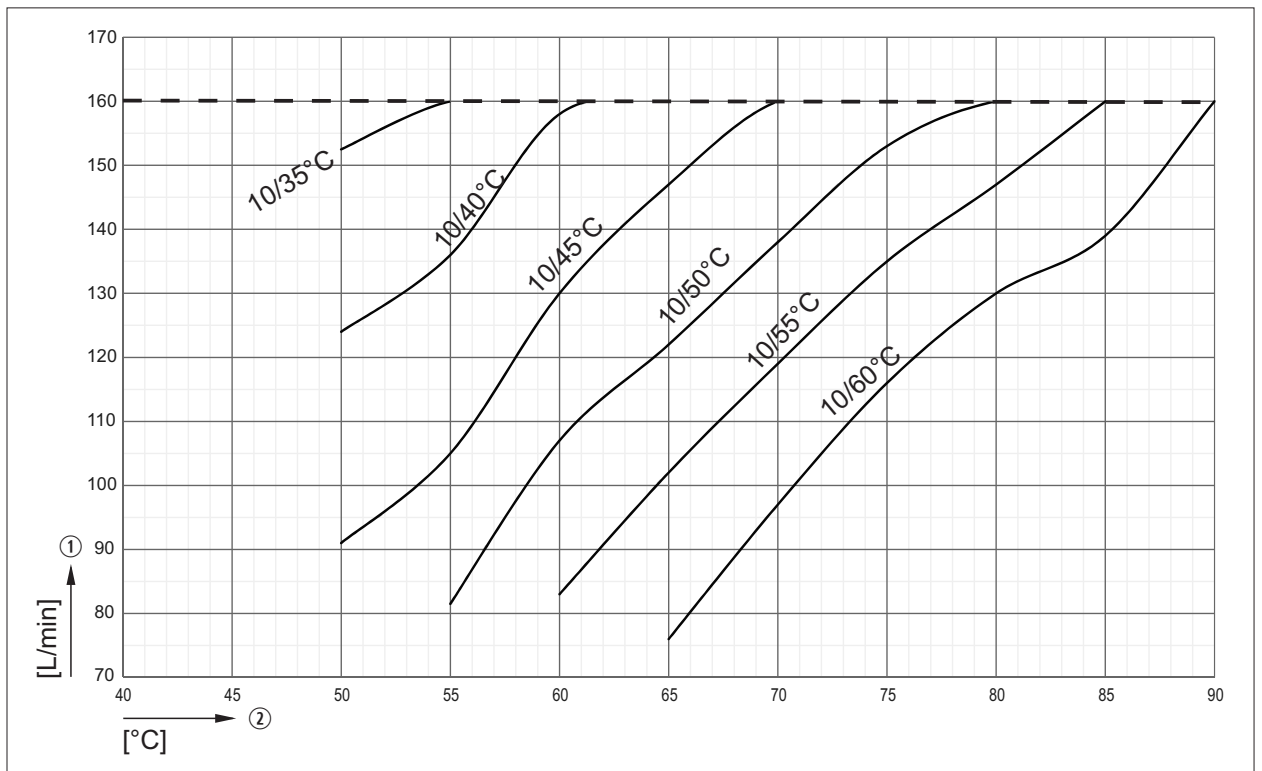
Abb. 6.6 Auslegungsdiagramm 4-er Kaskade
