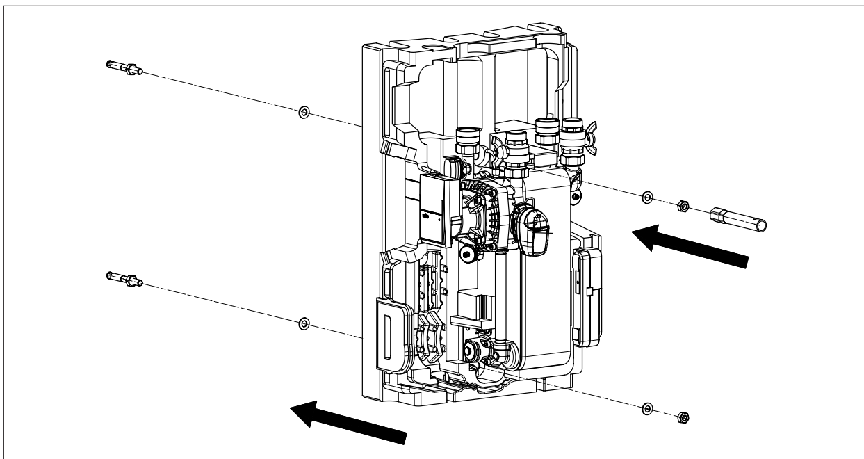
Abb. 3.3 Frischwasserstation montieren
