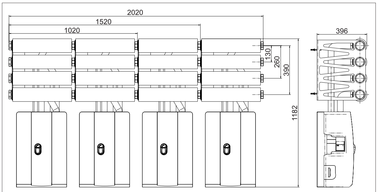
Abb. 5.1 Abmessungen
