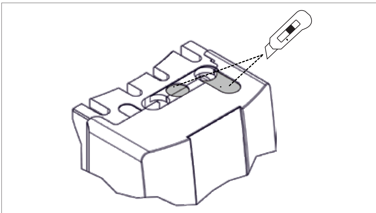
Abb. 3.4 Dämmung ausschneiden
