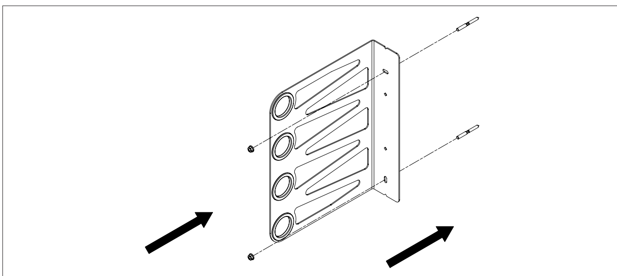
Abb. 3.7 Haltewinkel montieren
