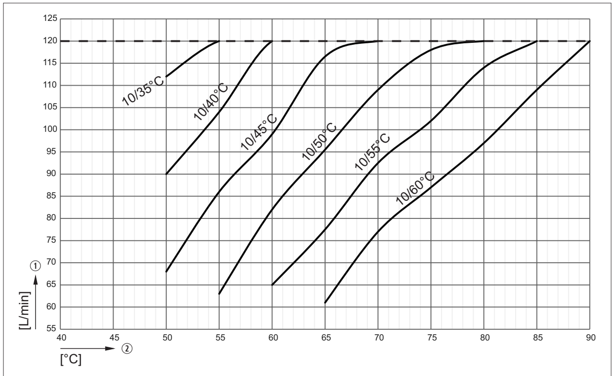
Abb. 6.5 Auslegungsdiagramm 3-er Kaskade
