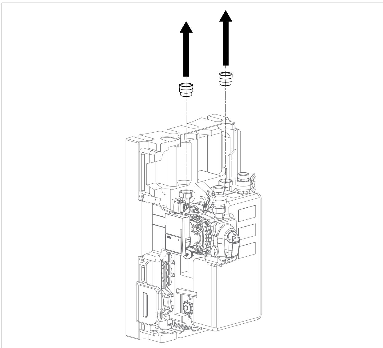
Abb. 3.5 Anschlüsse entfernen
