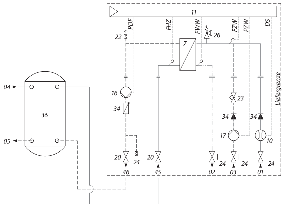
Prizipschaltbild
