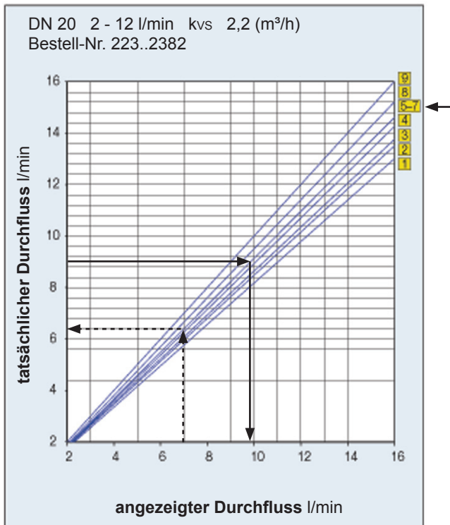
Diagramm 1: für Durchfluss-Regulierung DN20 2-12 l/min (bis 8 Kollektoren)
