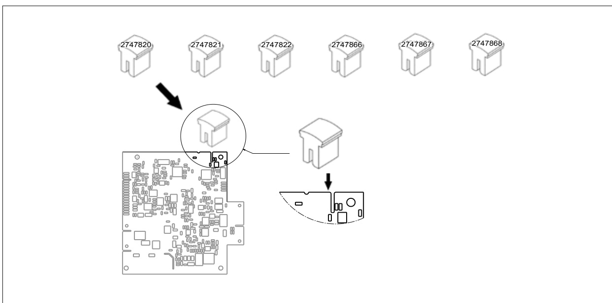
Abb. 4.7 Übersicht Parameterstecker
