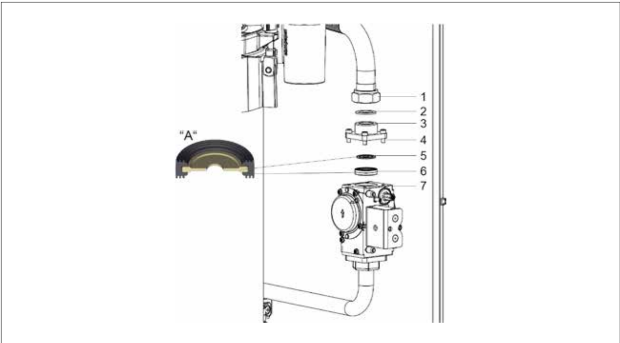
Abb. 4.1 Gasdrosselblende entnehmen
