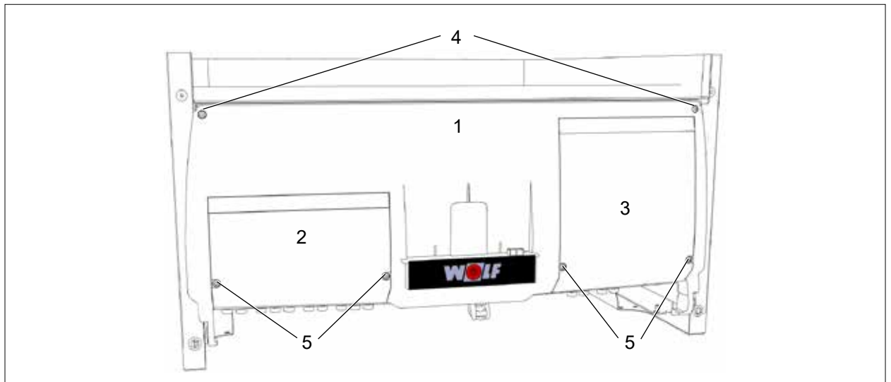
Abb. 4.8 Regelungsgehäuse schließen
