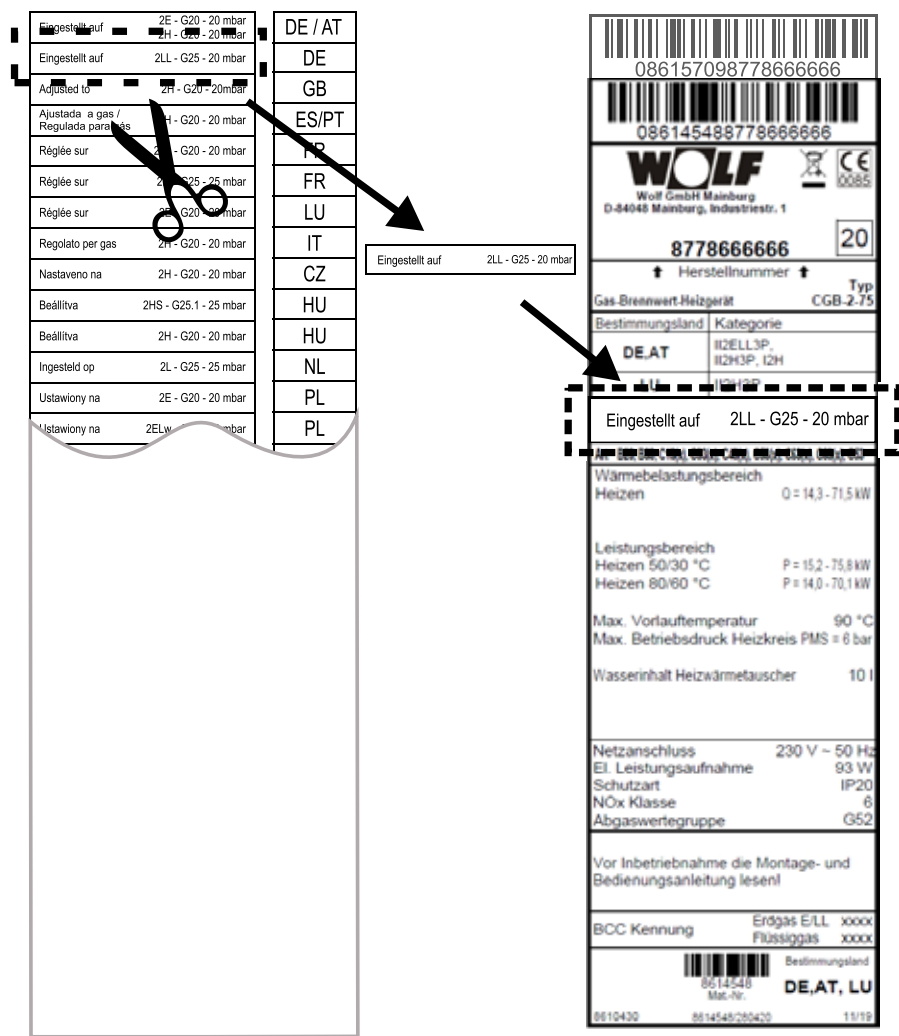
Abb. 4.3 Typenschild tauschen
