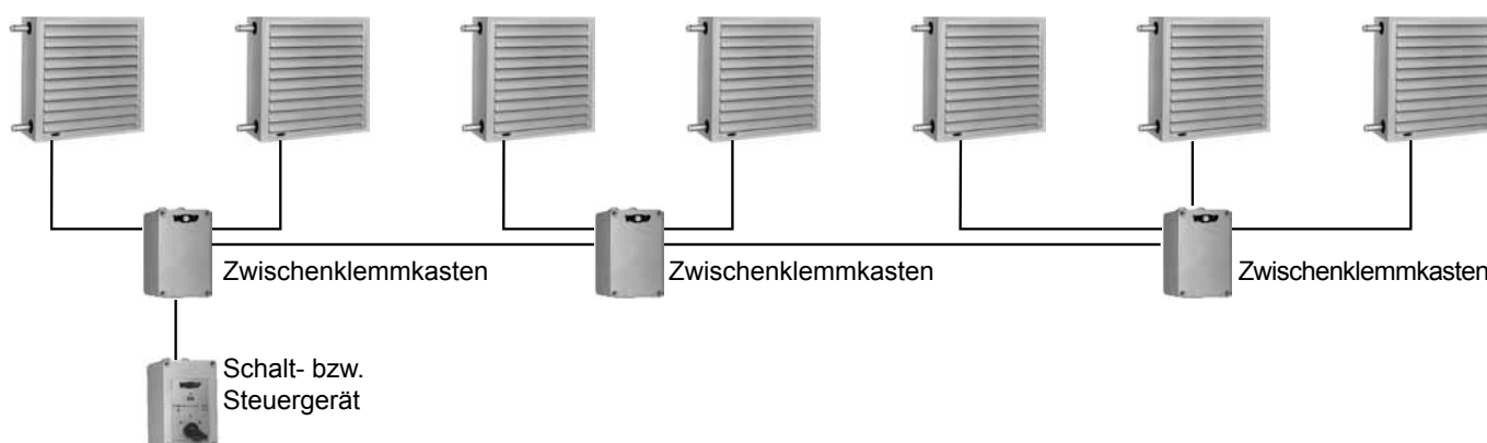
Anschluss von 7 LH-S-Geräten mit 3 Zwischenklemmkästen
