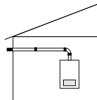
Luft-/Abgasführung waagrecht durch Außenwand C12x (Siehe Seite 16)
