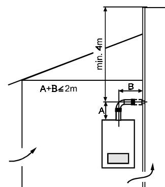
Anschluß an Abgasschornstein B32 (Siehe Seite 16)
