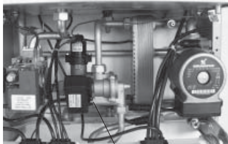
Einstellschraube
