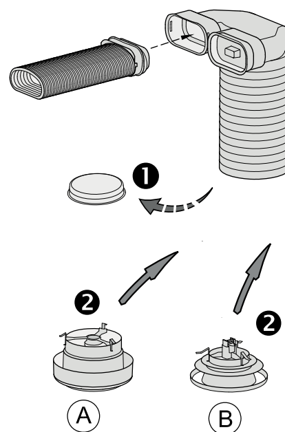
Rechtwinkliger Anschluss für die Montage der Ventile
