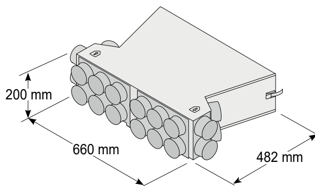
Luftverteiler System B
