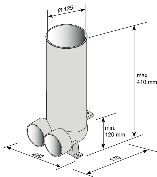
Anschlussstück für Ventil DN125
