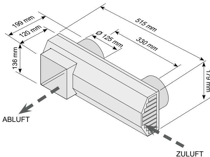
Doppelgitter
