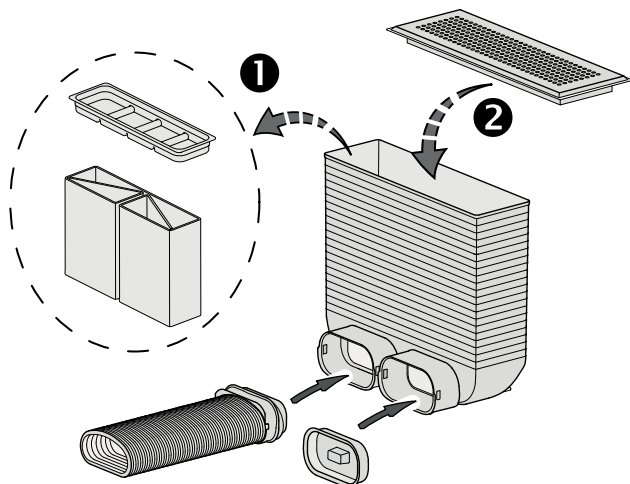
Rechtwinkliger Anschluss für die Montage des Bodengitters
