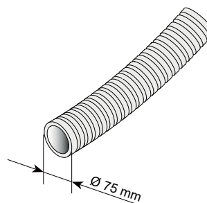
Luftverteilschlauch (Rolle 50 m)
