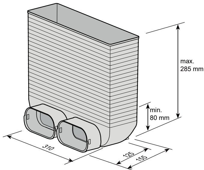
Anschlussstück Bodengitter
