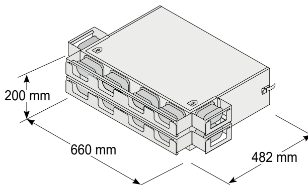
Luftverteiler System A
