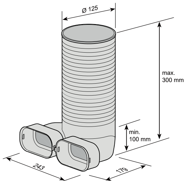
Anschlussstück für Ventil DN125
