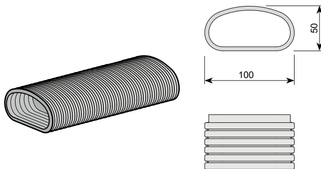
Luftverteilschlauch (Rolle 50 m)
