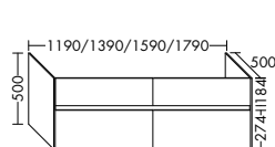
WXQQ119/139/159/179
