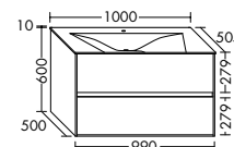
SGKG100
