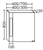
SPNF040/050/060/070 SPOB040/050/060/070*
