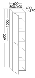
HSMS030/040/050/060 HSMT030/040/050/060
