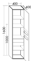
HSNZ040
