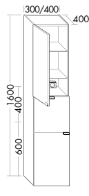
HSMW030/040
