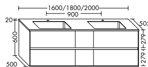
SGKF160/180/200
