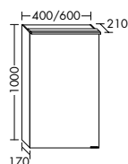
SPMZ040/060 SPNV040/060*
