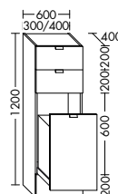
UHEO030/040/060
