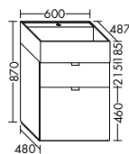
SFYF060
