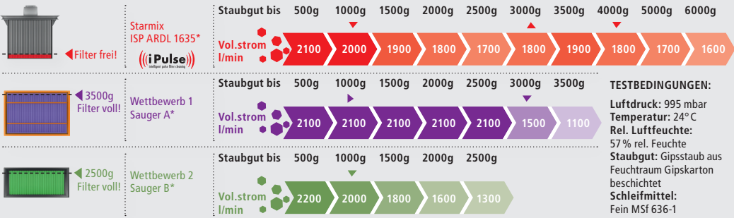
Füllstand-/Volumenstromvergleich mit Gipskarton
