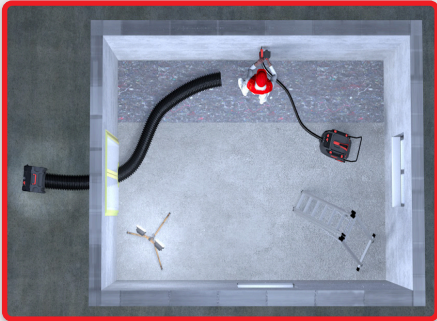
Zuluftschlauch im Raum. Gerät und gereinigte Abluft im Nebenraum. (Unterdruck-Betrieb)
