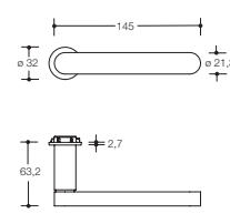
Nieuw Model 270XAM
