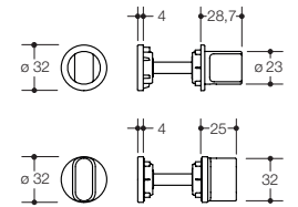
WC-rozet mini 306X...MNR, 306X...MNRHT
