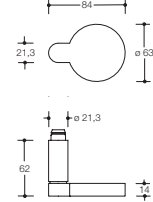
Nieuw Model 276X
