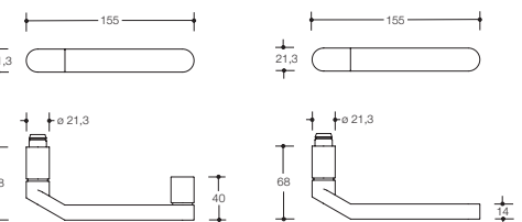
Nieuw Model 273X
