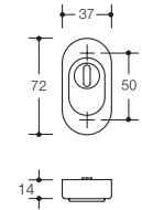
Veiligheidsrozet met cilinderbescherming 316...Z...
