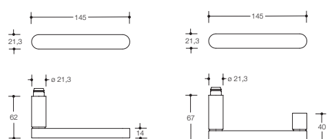
Nieuw Model 271X
