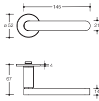
Nieuw Model 270PI....
