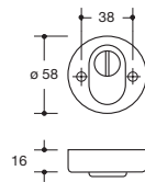
Veiligheidsrozet met cilinderbescherming 306...Z...
