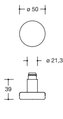
Modell 107X
