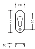
Schutzrosette 316X..ES...
