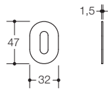
Schlüsselrosette mini 306XAM
