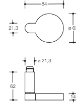
Neu Modell 276X
