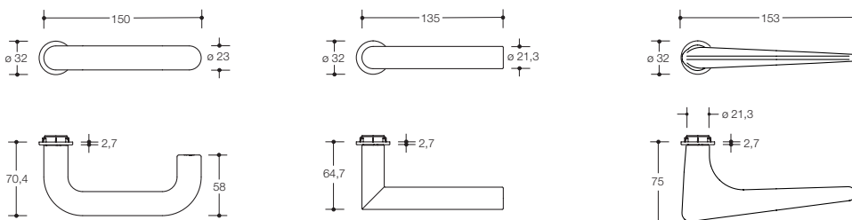
Modell 111...M
