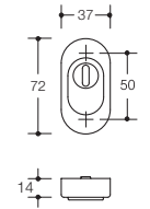
Schutzrosette mit Zylinderabdeckung 316...Z...
