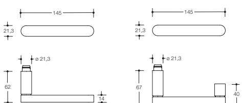
Neu Modell 271X
