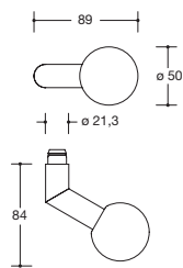
Modell 108X
