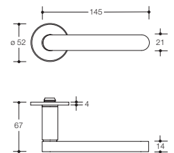
Modell 270PI....
