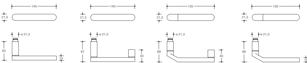
Modell 271X
