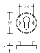
Schutzrosette 306.23X..ES...
