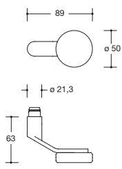
Modell 106X
