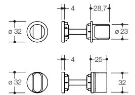
WC-Rosette mini 306X...MNR, 306X...MNRHT
