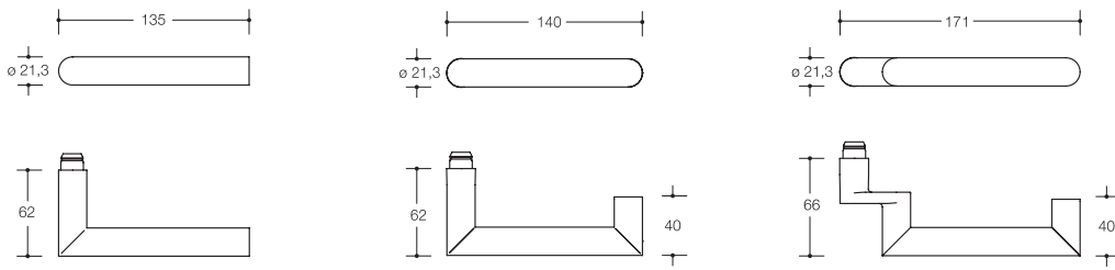
Modell 162.21P...
