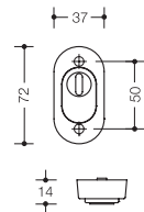
Schutzrosette 316X..ESZ
