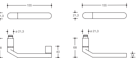
Neu Modell 273X
