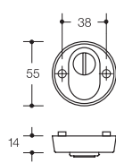
Schutzrosette 306.23X..ESZ...
