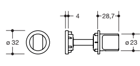
WC-Rosette 306P..MNR
