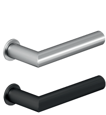
Türdrücker 162XAM06.230 Edelst. 162XPM06.230 Pulver Neu
