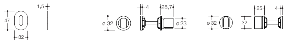
Schlüsselrosette mini 306XAM
