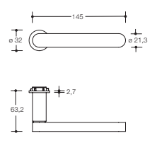
Neu Modell 270XAM
