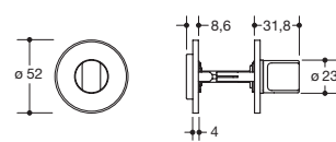
WC-Rosette 306..INR
