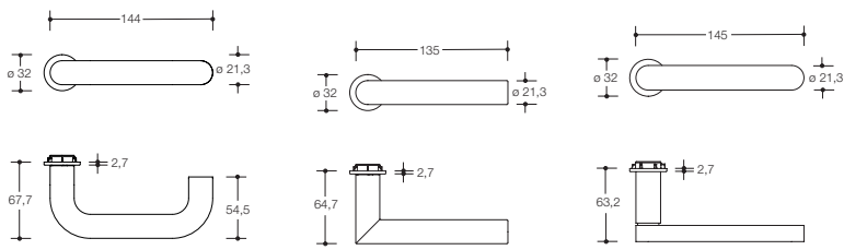
Modell 111XAM
