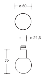
Modell 109X
