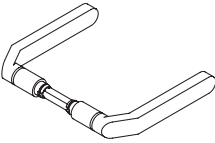
Rahmentürdrücker H-Technik, Klasse 4 274XVH 274XVHLT
