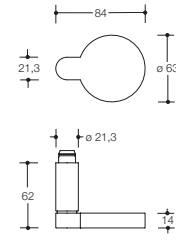
Modell 276X
