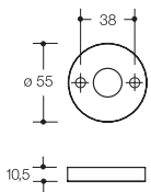
Drückerrosette 305...X..
