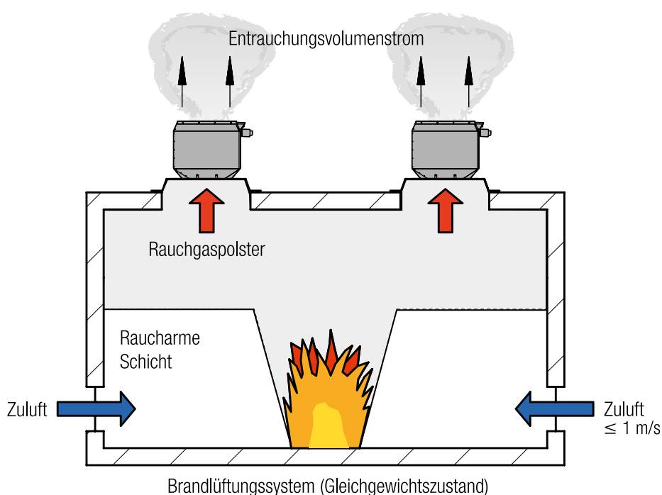
Bild 1 Gleichgewichtszustand zwischen zuströmender Luft und abgeführten Rauchgasen
