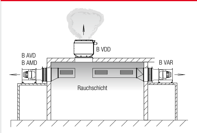
Bild 2 Ventilatoren außerhalb des Rauchabschnitts und außerhalb des Gebäudes
