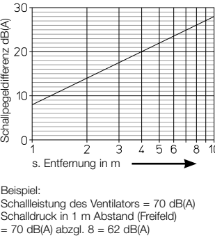
Bild 1 Differenz von Schallleistung zu Schalldruck mit der Entfernung
