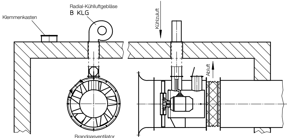
Bild 6 Aufstellung im Brandraum
