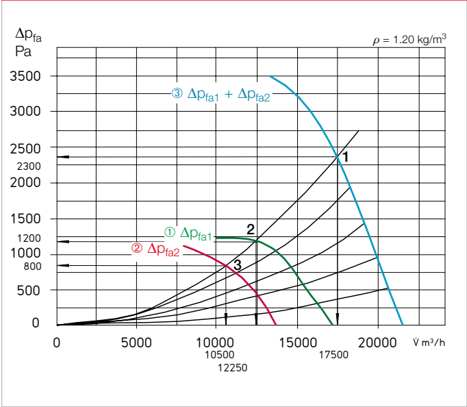
Kennlinie 1
