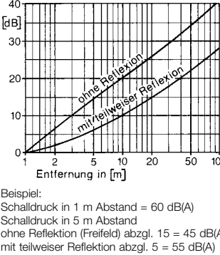
Bild 2 Schalldruckpegel-Abnahme mit der Entfernung
