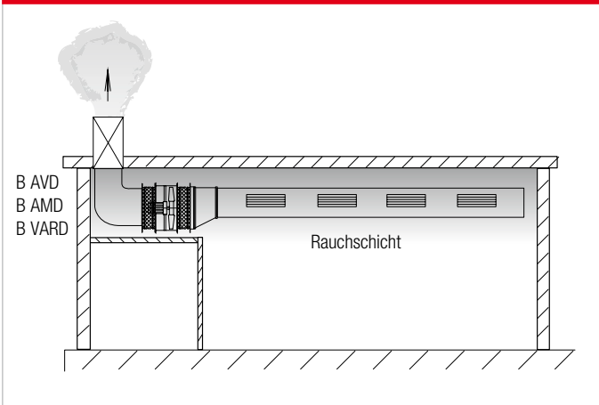
Bild 4 Ventilator innerhalb des Rauchabschnitts
