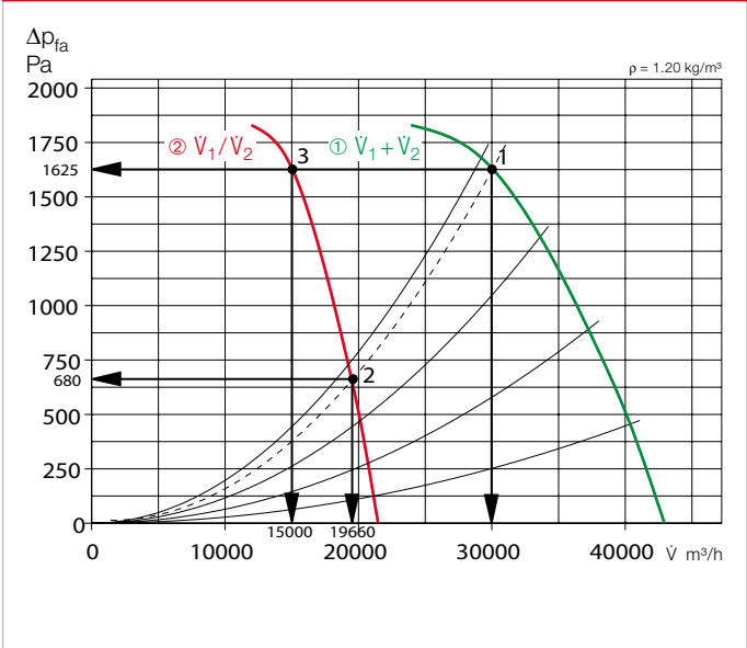
Kennlinie 2
