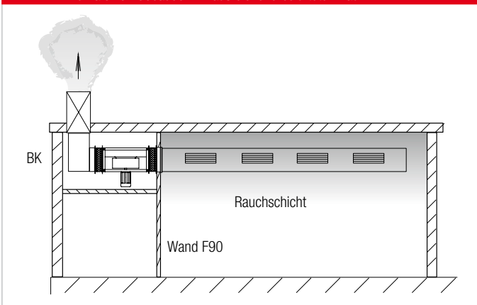
Bild 3 Ventilatoren außerhalb des Rauchabschnitts, innerhalb von Gebäuden im ausreichend belüfteten Raum
