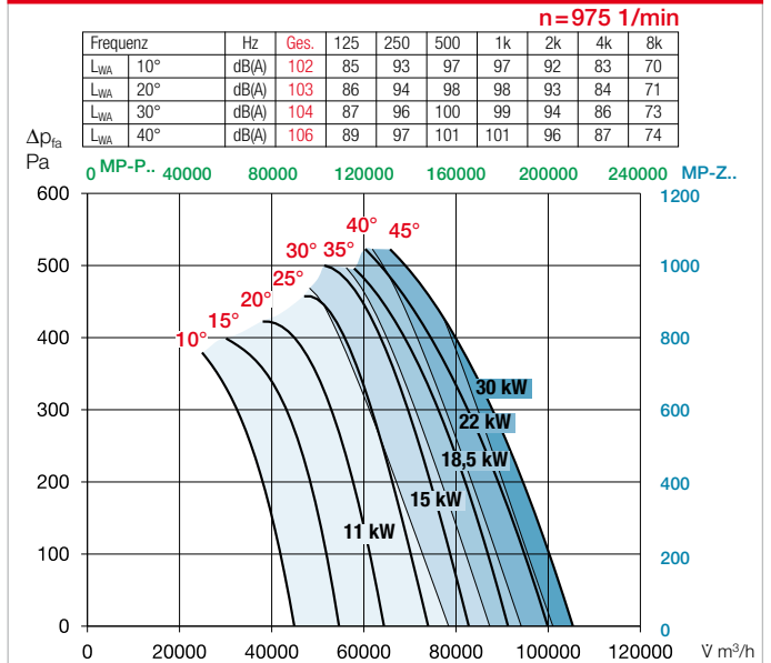
Kennlinien AMD / B AMD 1120/6
