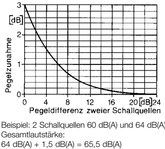
Bild 4 Addition mehrerer Schallquellen mit unterschiedlichen Schallpegeln
