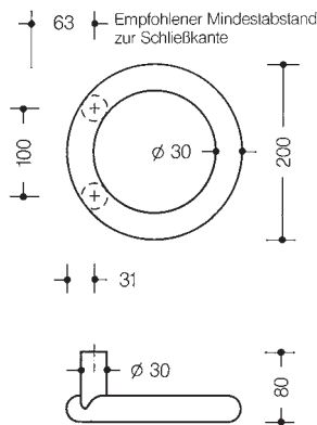
HEWI Griff ø 30 mm · aus hochwertigem Polyamid, Achsmaß 100 mm
