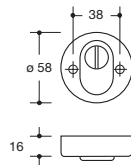
Schutzrosette mit Zylinderabdeckung 306...Z...
