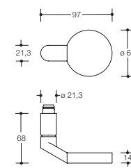
Modell 277X...
