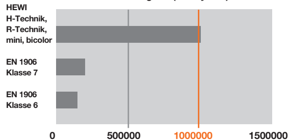
Dauerhaftigkeit (Prüfzyklen)
