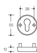
Schutzrosette 306.23X..ES...
