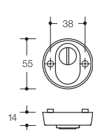
Schutzrosette 306.23X..ESZ...
