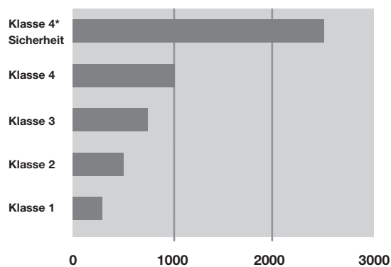
Zugfestigkeit
