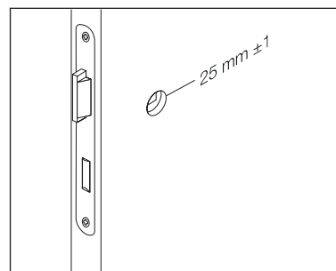
Fräsmaß | Türdrücker
