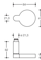
Modell 276X...
