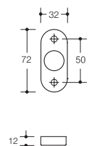
Drückerrosette 315...X
