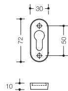
Schutzrosette 316X..ES
