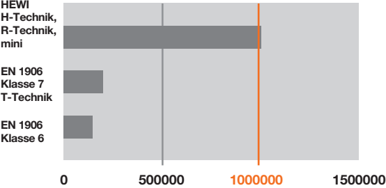
Dauerhaftigkeit (Prüfzyklen)
