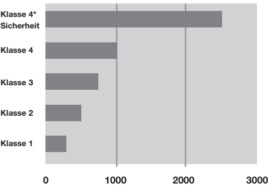
Zugfestigkeit
