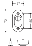
Schutzrosette 316X..ESZ
