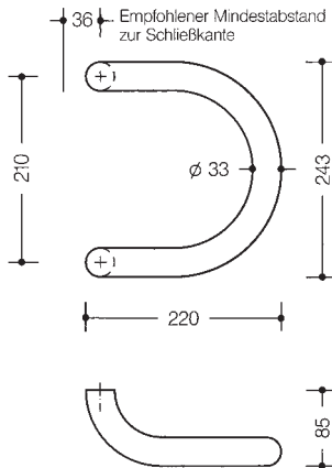
HEWI Griff ø 33 mm · aus hochwertigem Polyamid, Achsmaß 210 mm Besonders geeignet für Rahmentüren gemäß DGUV (siehe Seite 201).
