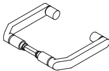
Rahmentürdrücker H-Technik, Klasse 4 273XVH 273XVHLT
