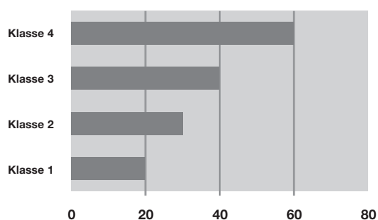
Torsiesterkte
