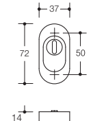
Veiligheidsrozet met cilinderbescherming 316...Z...
