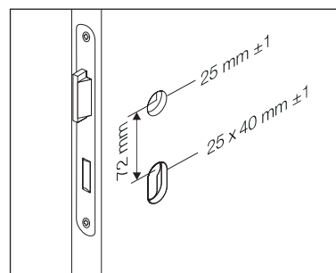
Freesmaat | Profielcilinder of baardsleutel
