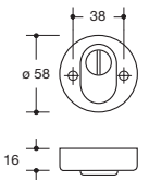
Veiligheidsrozet met cilinderbescherming 306...Z...
