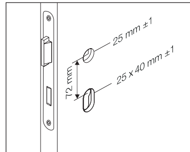
Freesmaat | Profielcilinder of baardsleutel
