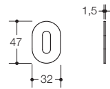
Sleutelrozet mini 306XAM
