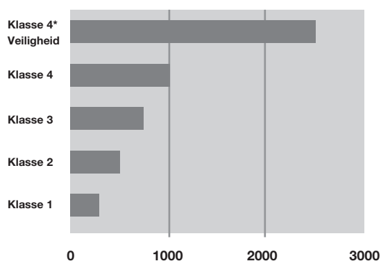
Treksterkte
