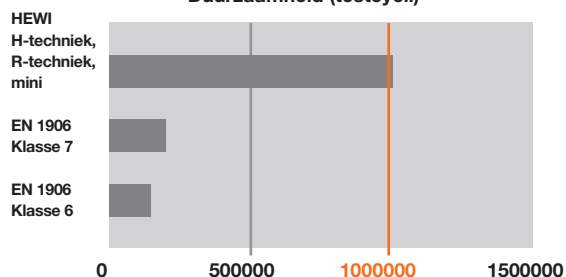
Duurzaamheid (testcycli)
