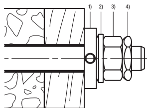
Vorsteckmontage mit FIS A und Injektionssystem Größen: M12, M16, M20, M24
